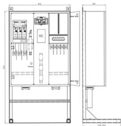
Beispiel Ansicht BAK 250 A
