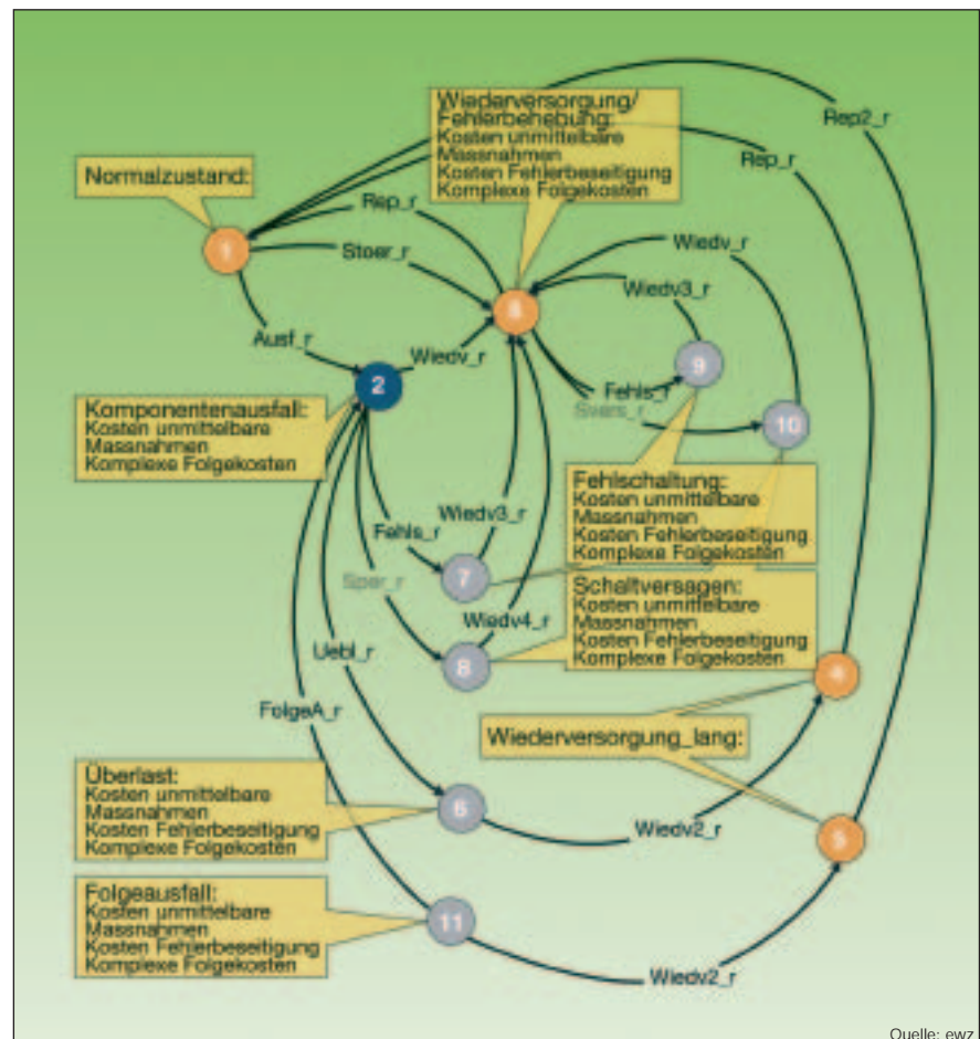
Bild 8 Zustandsdiagramm für Einfachausfälle von Komponenten im Unterwerk
