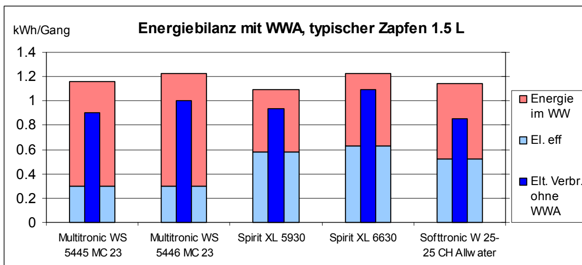
Fig. 3.1 Waschmaschinen mit Warmwasseranschluss: Energieverbrauchsrechnung mit Zapfen 1.5 L
