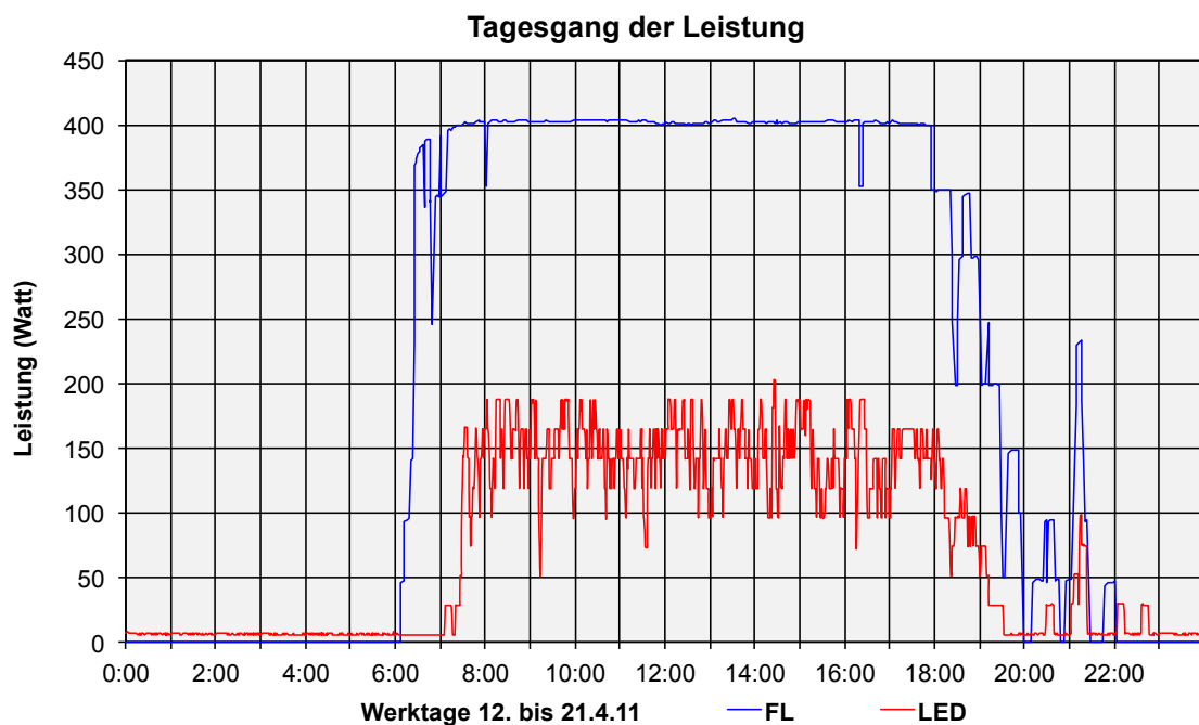
Abbildung 9: Mittelwertkurven der Leistung an Werktagen in der 1. Messperiode
