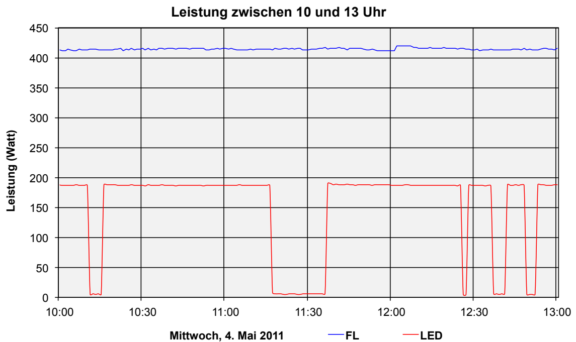
Abbildung 13: Leistung zwischen 10 und 13 Uhr an einem typischen Werktag in der 2. Messperiode
