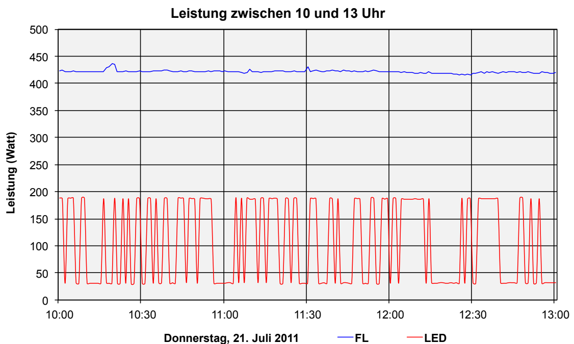
Abbildung 17: Leistung zwischen 10 und 13 Uhr an einem typischen Werktag in der 4. Messperiode
