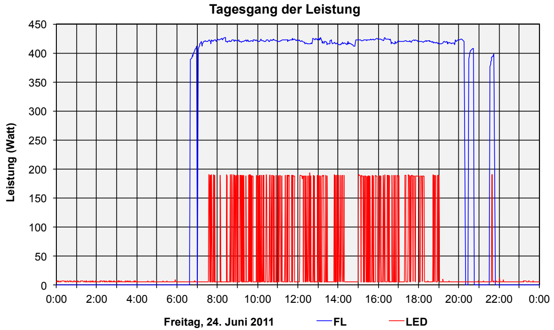
Abbildung 14: Tagesgang der Leistung an einem typischen Werktag in der 3. Messperiode
