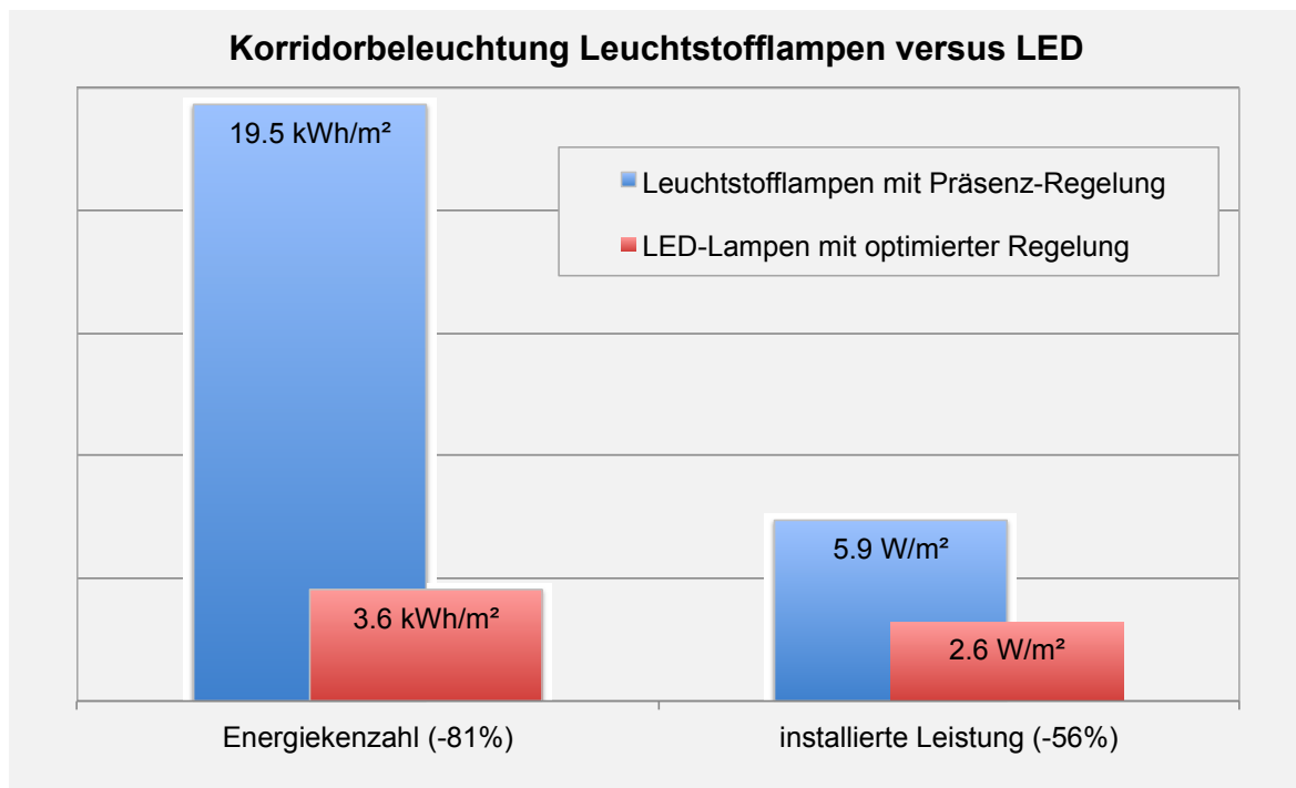
Abbildung 1: Korridorbeleuchtung Leuchtstofflampen versus LED
