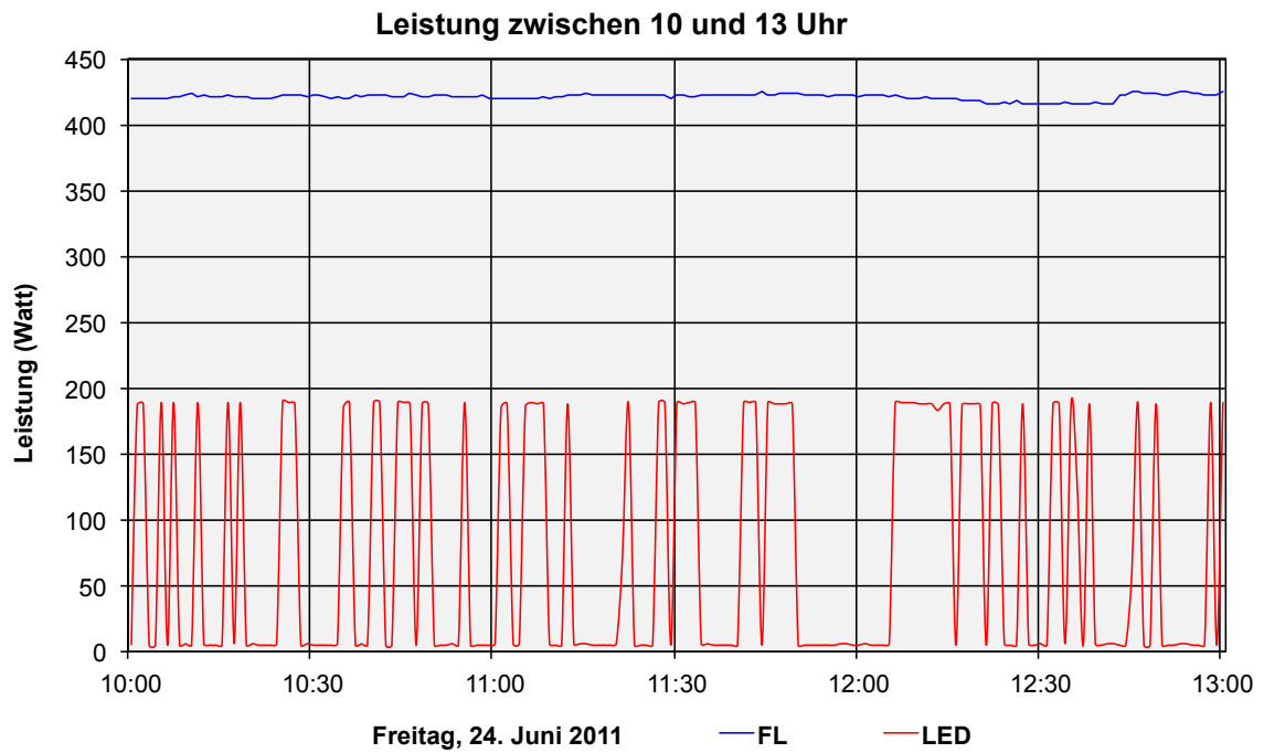
Abbildung 15: Leistung zwischen 10 und 13 Uhr an einem typischen Werktag in der 3. Messperiode
