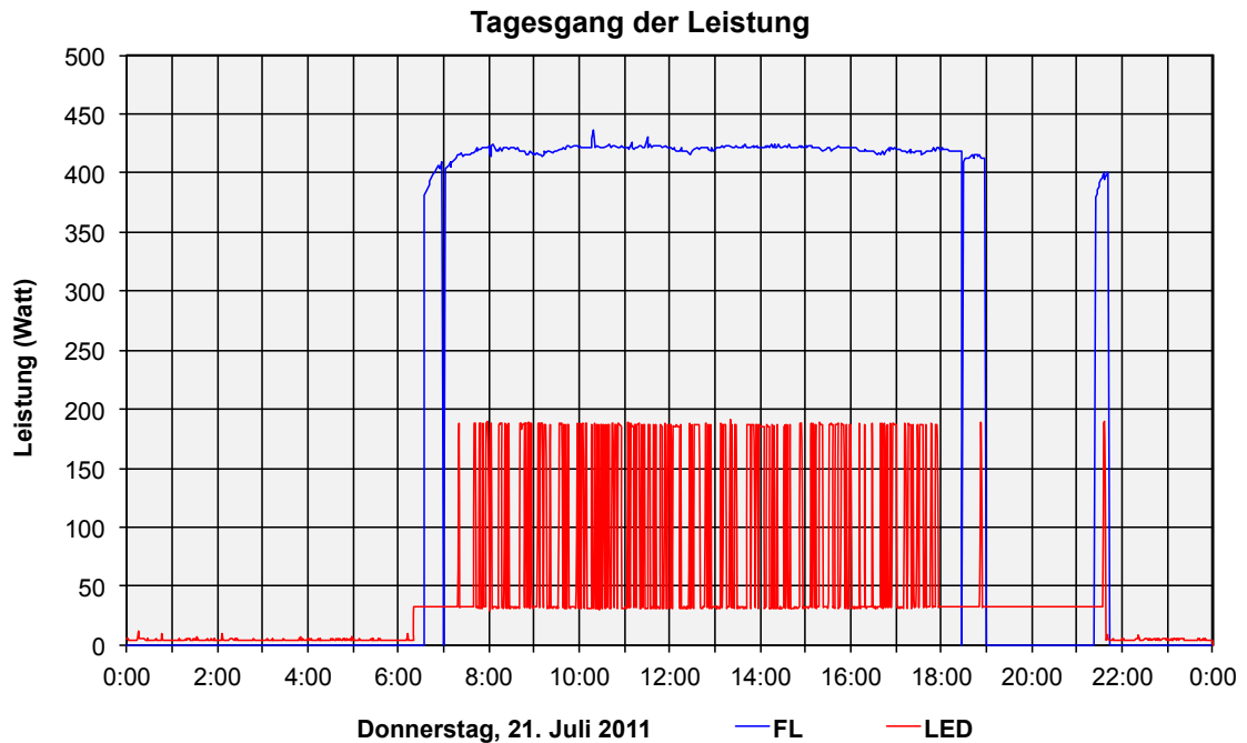
Abbildung 16: Tagesgang der Leistung an einem typischen Werktag in der 4. Messperiode
