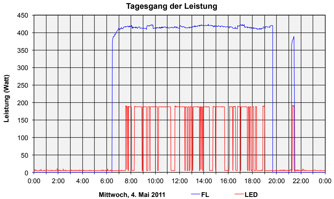
Abbildung 12: Tagesgang der Leistung an einem typischen Werktag in der 2. Messperiode
