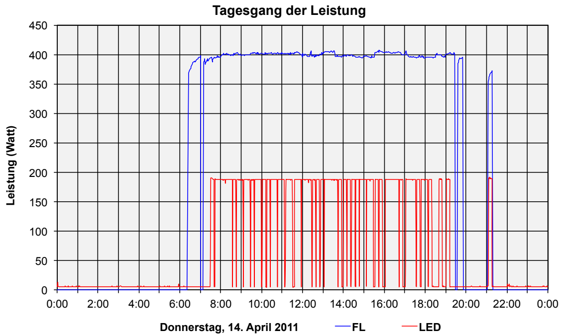
Abbildung 10: Tagesgang der Leistung an einem typischen Werktag in der 1. Messperiode
