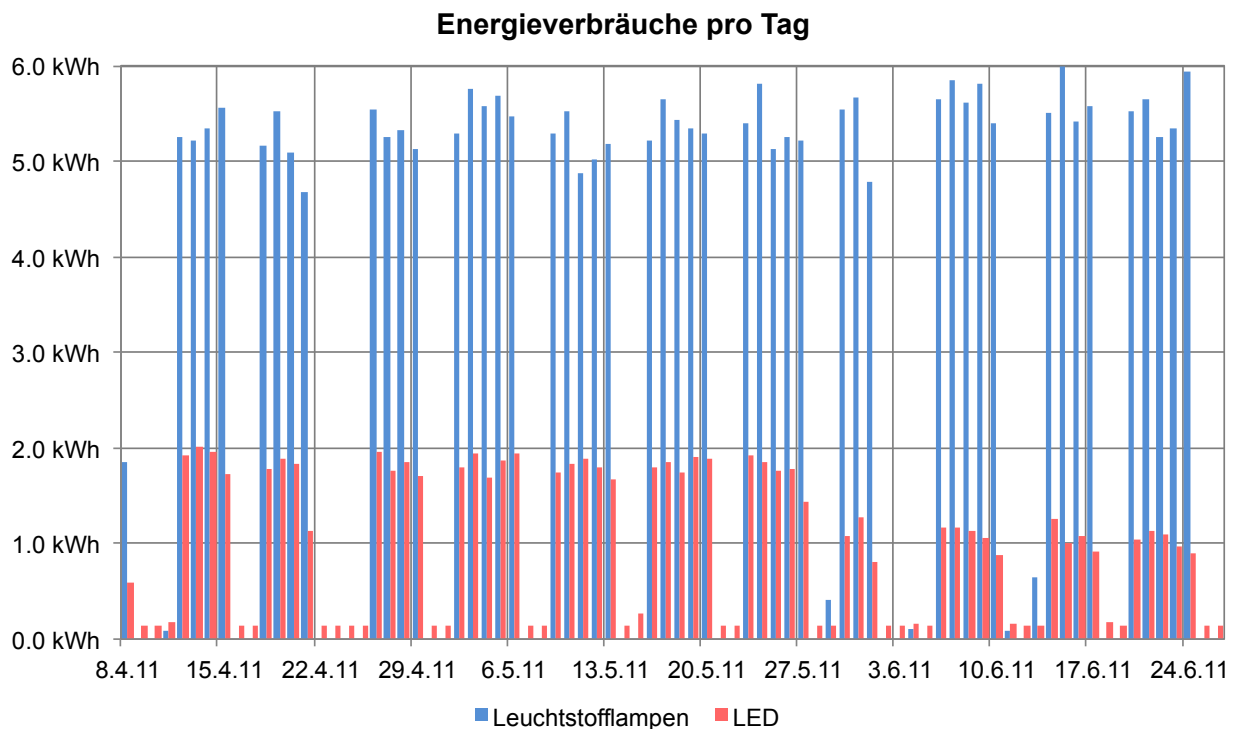
Abbildung 8: Tägliche Energieverbräuche während den ersten drei Messperioden
