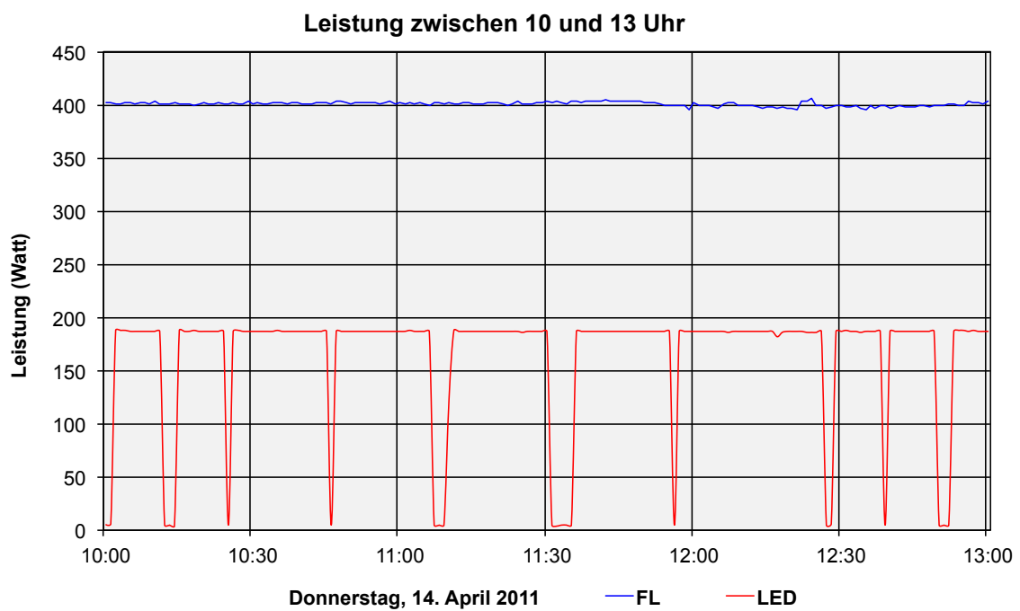
Abbildung 11: Leistung zwischen 10 und 13 Uhr an einem typischen Werktag in der 1. Messperiode
