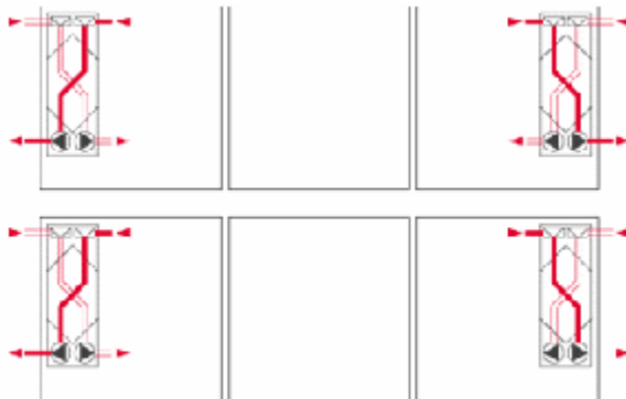
Figur 51: Einzelraum-Komfortlüftung (Quelle: MINERGIE)
