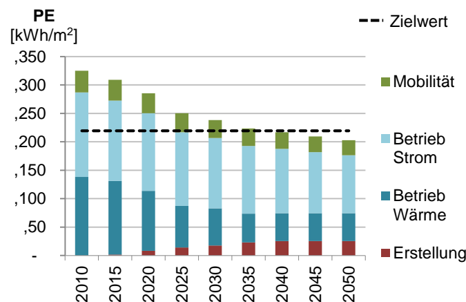
Figur 2: Übersicht Portfolioentwicklung 2010-2050 Primärenergie gesamt
