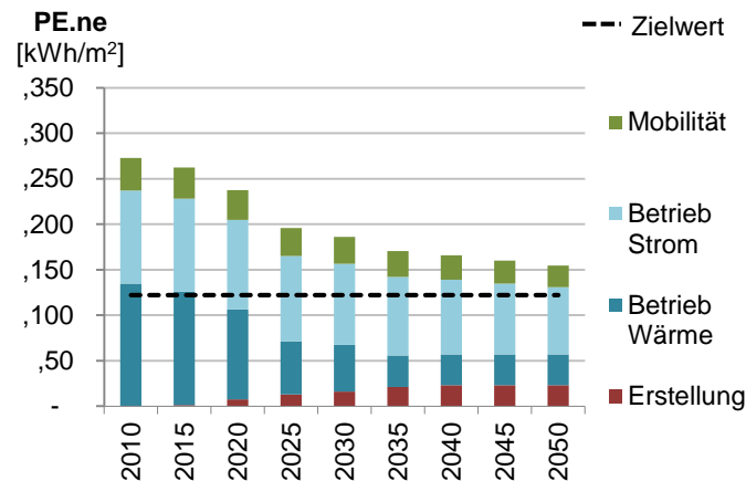
Figur 1: Übersicht Portfolioentwicklung 2010-2050 Primärenergie nicht erneuerbar
