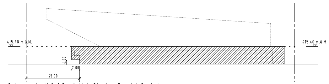
Schemaschnitt 2-2 Baufeld A, Stadion, Bereich Sockel
