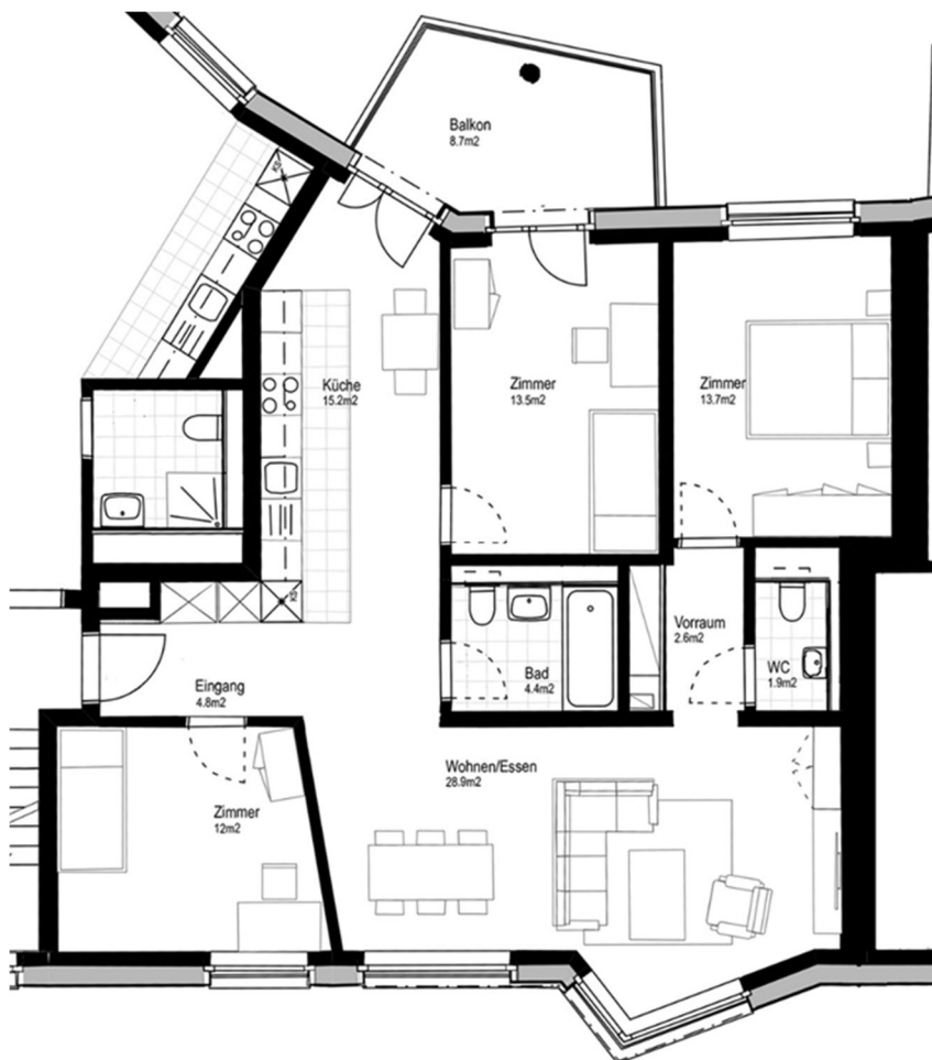
Standard-4,5-Zimmer-Wohnung, 97 m 2
