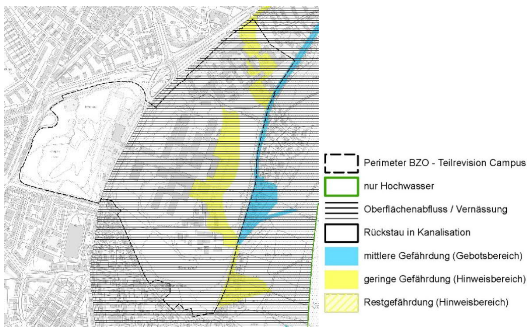
Abb. 20: Naturgefahren, Hochwasser
