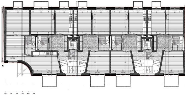
Grundrissplan 1. Obergeschoss
