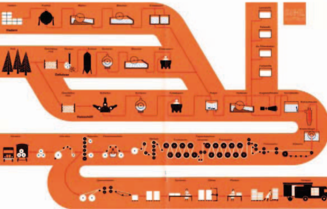
«Schematische Darstellung des Werdeganges des Papiers». Aus einer Werbebroschüre der Zürcher Papierfabrik an der Sihl, 1974. (StArZH, Bibliothekssignatur Db 788 Beil.)
