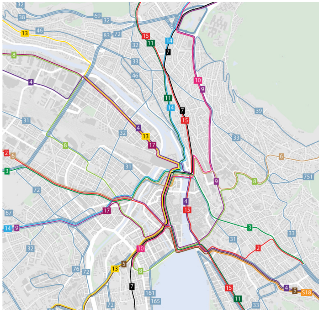
Abbildung 35: Liniennetzplan-Ausschnitt Teilraum Mitte für kurzfristige Angebotsmas- nahmen ohne grössere Infrastrukturanpas- sungen in Etappe 1
