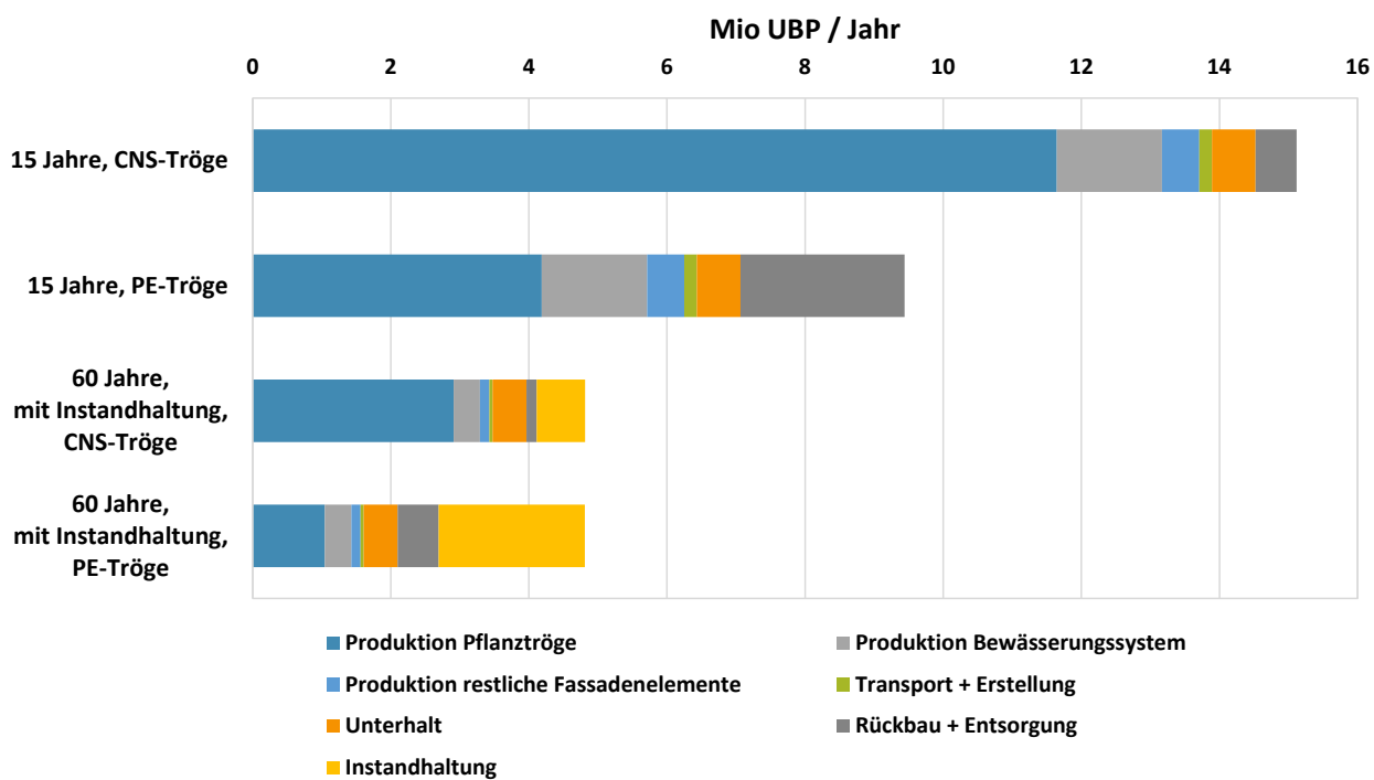
Abbildung 8: Gesamtumweltbelastung in Mio UBP pro Jahr, für eine Fassadenbegrünung mit einer Betriebsdauer von 15 Jahren sowie einer Betriebsdauer von 60 Jahren. Pro Betriebsdauer ist jeweils ein Szenario mit CNS- und PE-Pflanztrögen dargestellt, unterteilt in die verschiedenen Prozesse.
