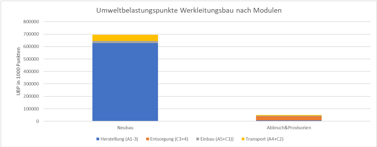
Abbildung 112: Mühlezellstrasse Werkleitungen:Umweltbelastungspunkte unterschieden nach Modulen
