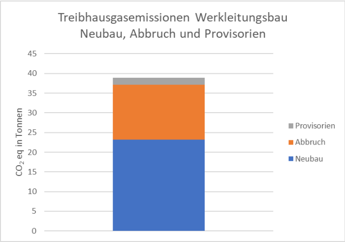
Abbildung 242: Universitätsstrasse Werkleitungen: Treibhausgasemissionen Neubau, Abbruch und Provisorien
