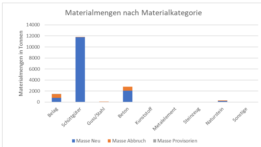
Abbildung 1: Allenmoosstrasse: Materialmengen nach Materialkategorien: Belag (Asphalt), Schüttgüter (Kiessande und Aushub), Guss/Stahl (Schachtdeckel und Schienen), Beton, Kunststoff (Rohre), Metallelemente (nur bei Sonderbauwerken), Steinzeug (Rohre), Naturstein (Randsteine und Pflasterung) und sonstige.
