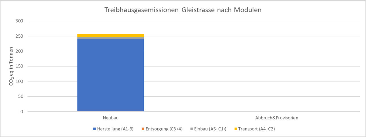
Abbildung 243: Universitätsstrasse Gleisbau: Treibhausgasemissionen unterschieden nach Modulen
