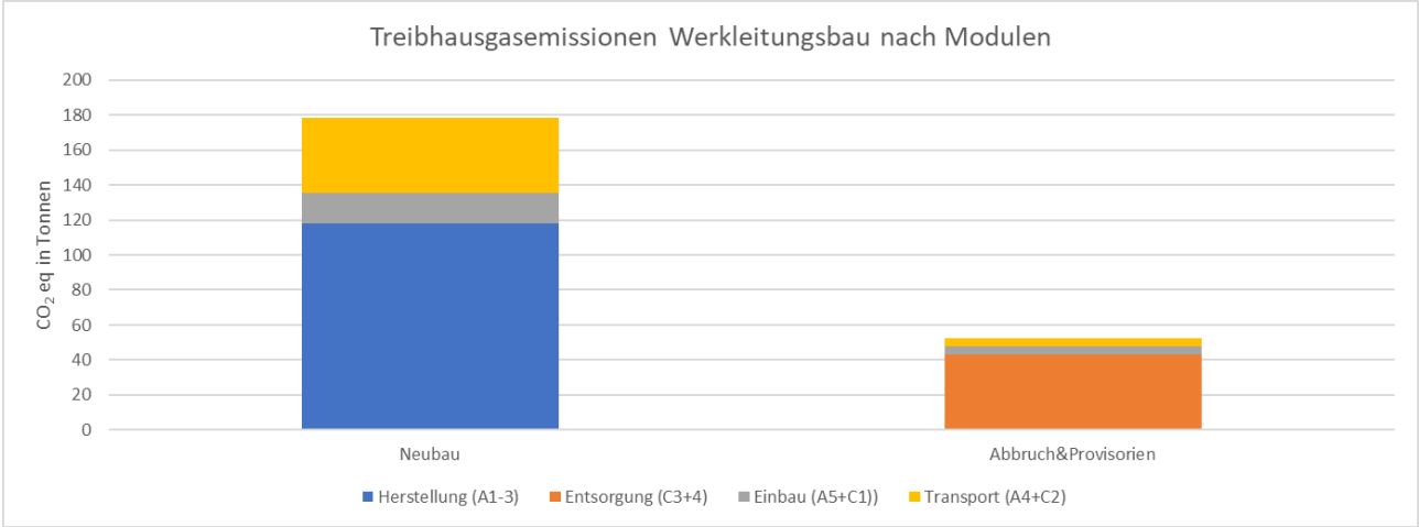
Abbildung 210: Wiesliacher Trichtenstrasse Werkleitungen: Treibhausgasemissionen unterschieden nach Modulen
