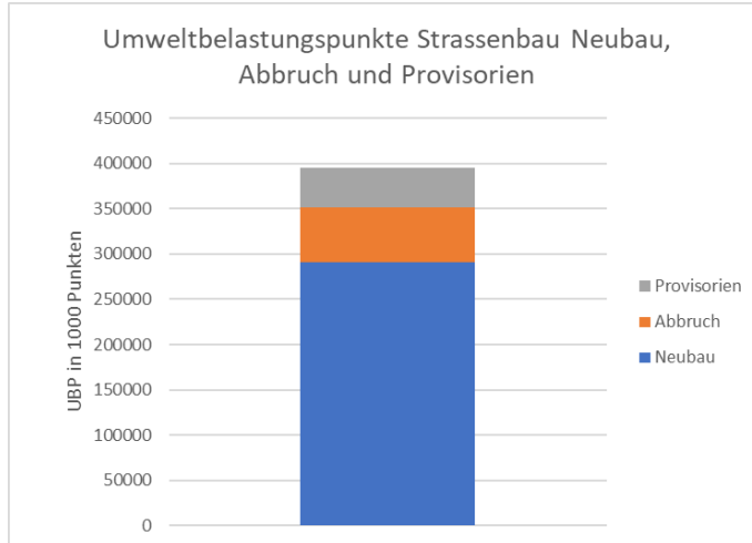
Abbildung 249: Universitätsstrasse Strassenbau: Umweltbelastungspunkte Neubau, Abbruch und Provisorien
