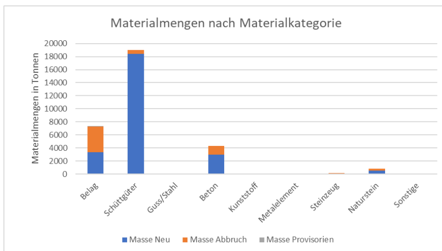
Abbildung 70: Manessestrasse: Materialmengen nach Materialkategorien: Belag (Asphalt), Schüttgüter (Kiessande und Aushub), Guss/Stahl (Schachtdeckel und Schienen), Beton, Kunststoff (Rohre), Metallelemente (nur bei Sonderbauwerken), Steinzeug (Rohre), Naturstein (Randsteine und Pflasterung) und sonstige.
