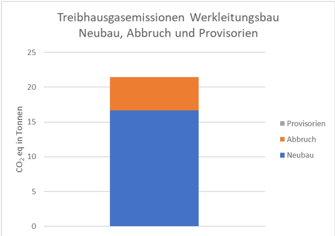
Abbildung 23: Gloriatrasse Werkleitungen: Treibhausgasemissionen Neubau, Abbruch und Provisorien
