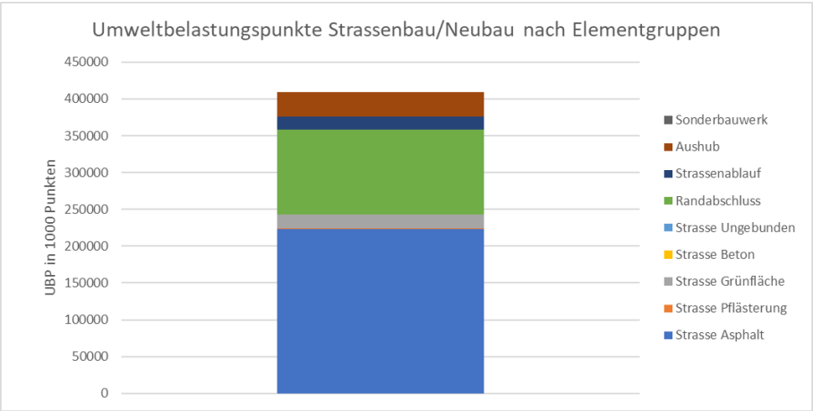
Abbildung 65: In der Ey Strassenbau: Umweltbelastungspunkte des Neubaus unterschieden nach Elementgruppen
