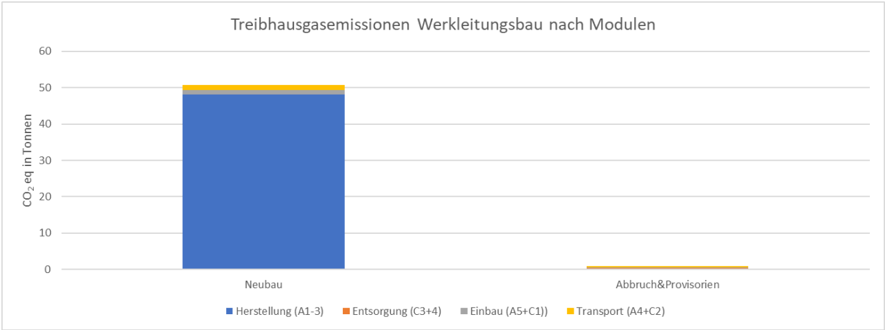
Abbildung 261: Winterthurerstrasse Werkleitungen:Treibhausgasemissionen unterschieden nach Modulen
