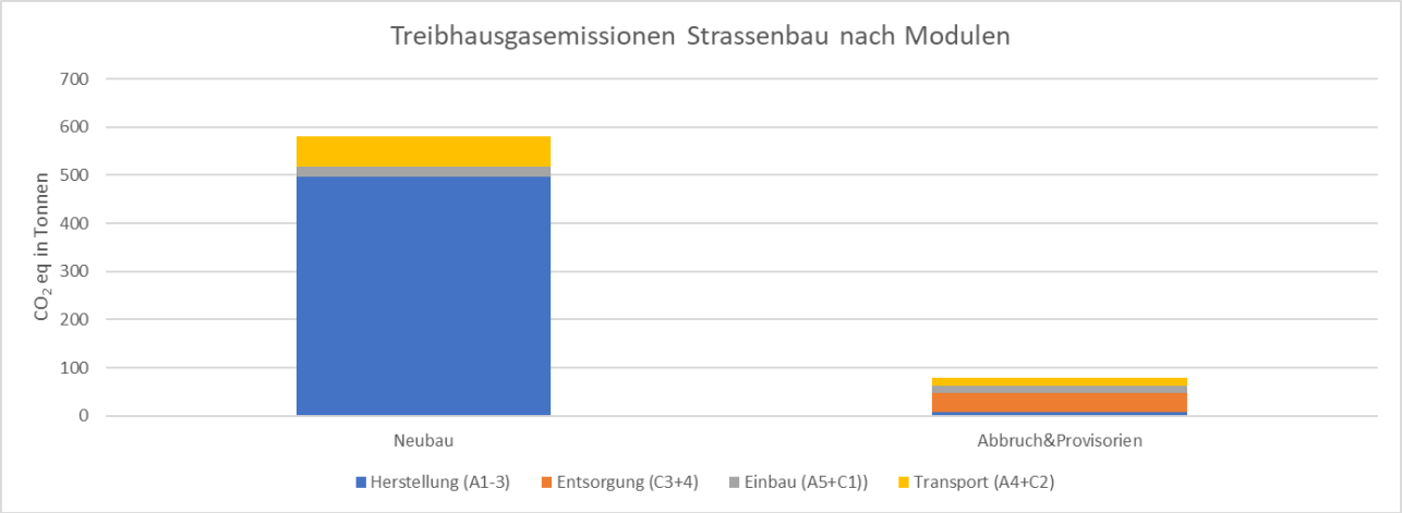
Abbildung 72: Manessestrasse Strassenbau: Treibhausgasemissionen unterschieden nach Modulen
