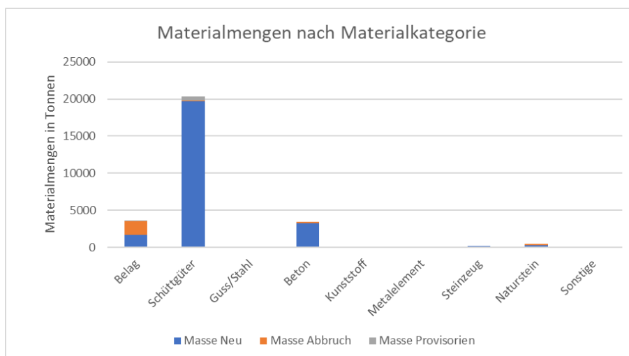
Abbildung 40: Haldenbach: Materialmengen nach Materialkategorie: Belag (Asphalt), Schüttgüter (Kiessande und Aushub), Guss/Stahl (Schachtdeckel und Schienen), Beton, Kunststoff (Rohre), Metallelemente (nur bei Sonderbauwerken), Steinzeug (Rohre), Naturstein (Randsteine und Pflasterung) und sonstige.
