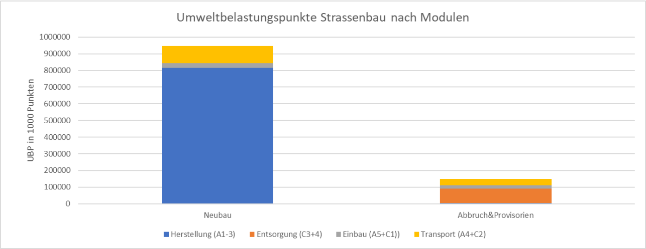
Abbildung 139: Regensburgstrasse: Umweltbelastungspunkte unterschieden nach Modulen
