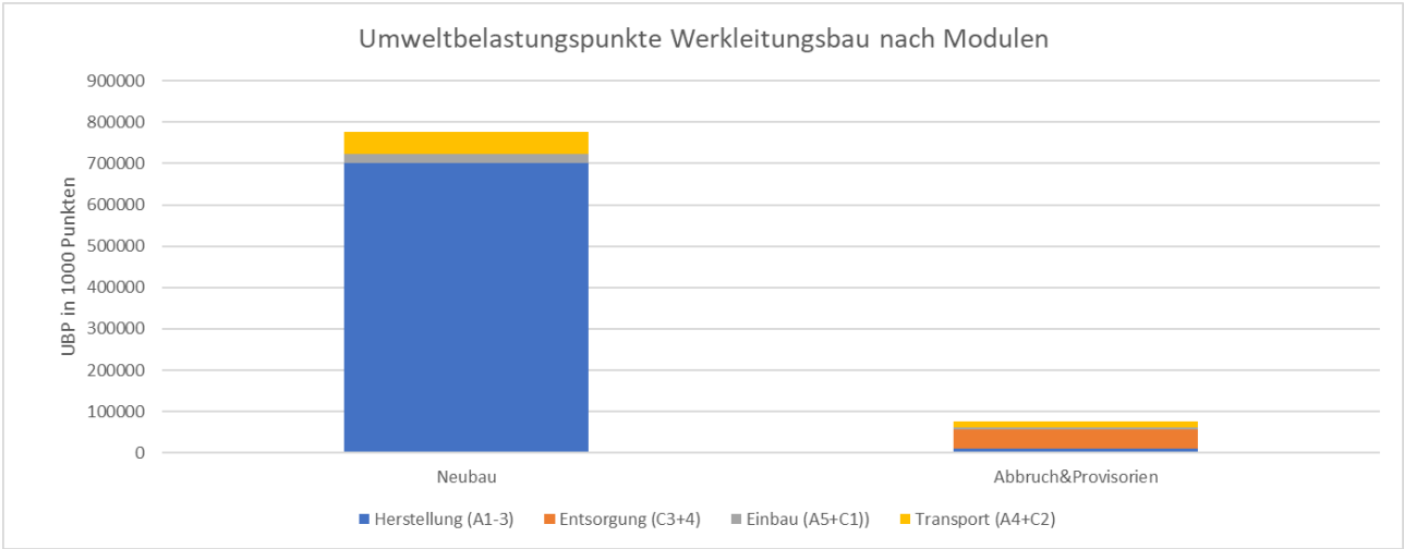
Abbildung 82: Manessestrasse Werkleitungen:Umweltbelastungspunkte unterschieden nach Modulen
