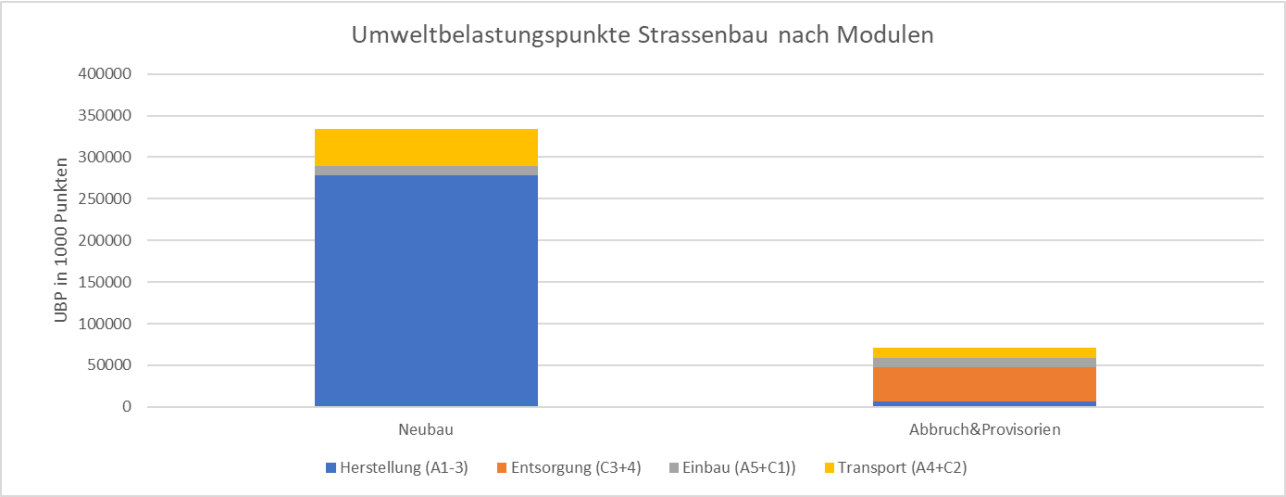
Abbildung 109: Mühlzellstrasse: Umweltbelastungspunkte unterschieden nach Modulen
