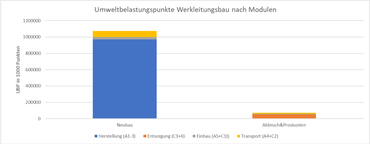
Abbildung 187: Sempacherstrasse Werkleitungen:Umweltbelastungspunkte unterschieden nach Modulen
