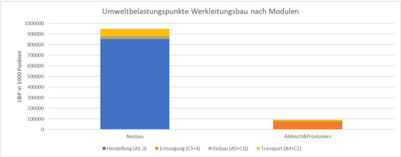
Abbildung 13: Allenmoosstrasse Werkleitungen:Umweltbelastungspunkte unterschieden nach Modulen
