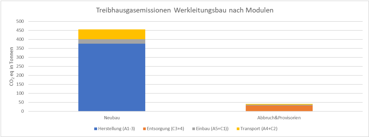
Abbildung 225: Witikonerstrasse Werkleitungen: Treibhausgasemissionen unterschieden nach Modulen
