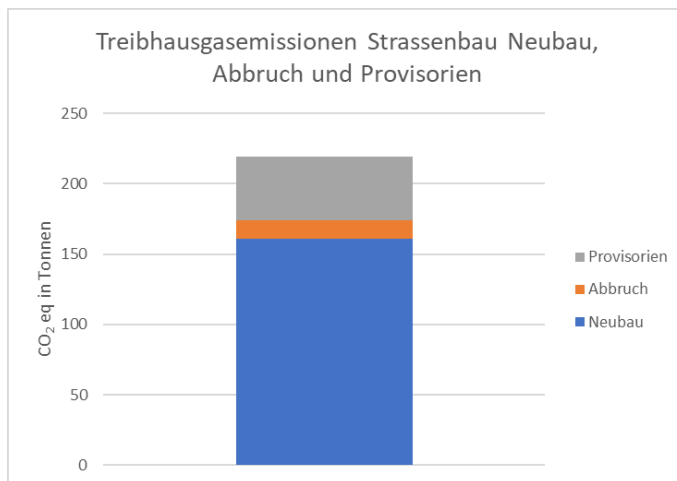
Abbildung 20: Gloriatrasse Strassenbau: Treibhausgasemissionen Neubau, Abbruch und Provisorien
