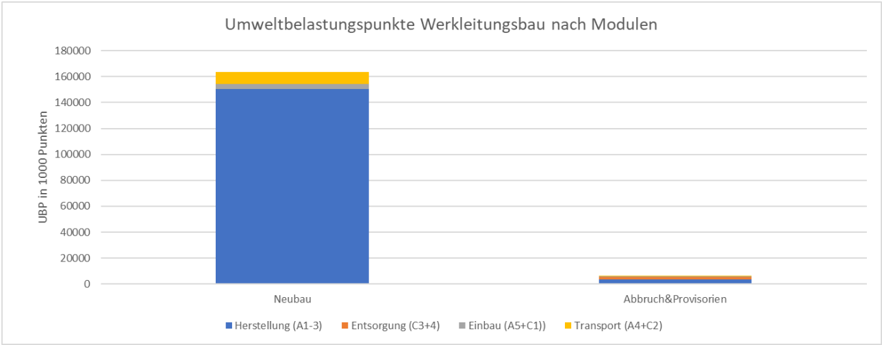
Abbildung 157: Rüdiger Staffel Werkleitungen:Umweltbelastungspunkte unterschieden nach Modulen
