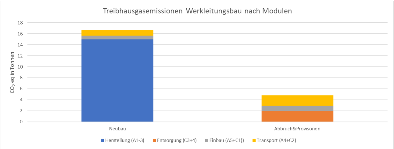
Abbildung 24: Gloriatrasse Werkleitungen: Treibhausgasemissionen unterschieden nach Modulen
