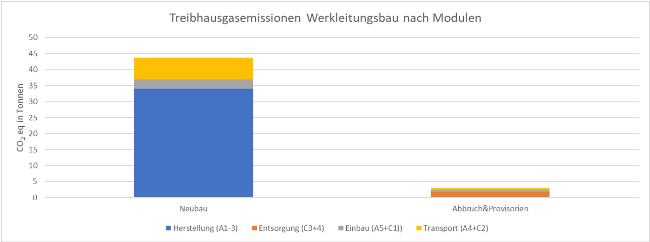
Abbildung 90: Marktplatz Oerlikon Werkleitungen:Treibhausgasemissionen unterschieden nach Modulen
