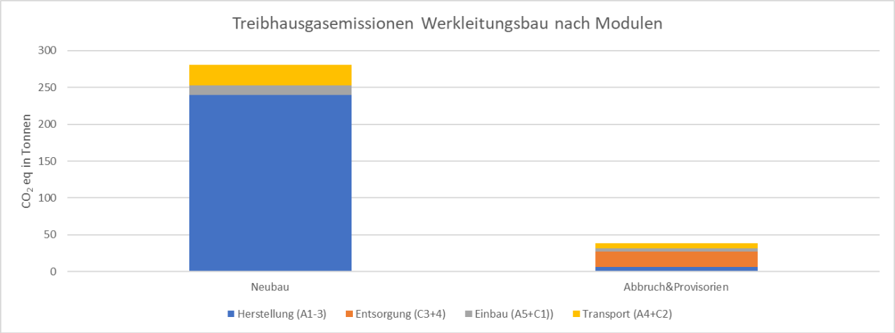
Abbildung 75: Manessestrasse Werkleitungen: Treibhausgasemissionen unterschieden nach Modulen
