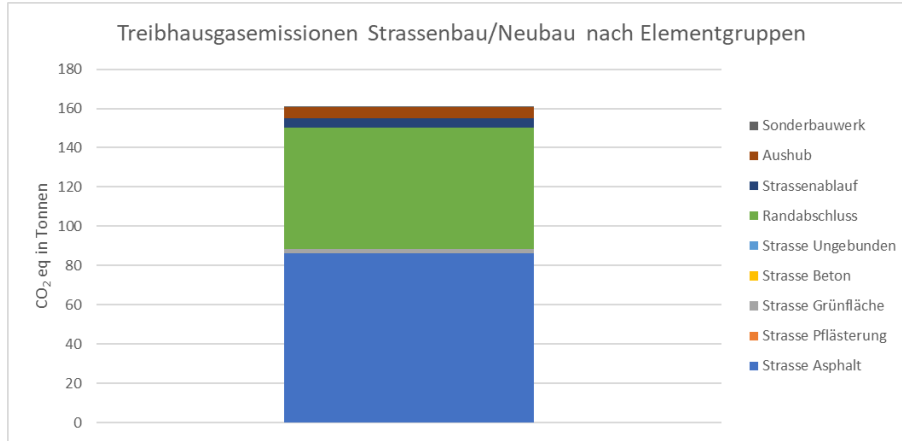
Abbildung 19: Gloriatrasse Strassenbau: Treibhausgasemissionen des Neubaus unterschieden nach Elementgruppen
