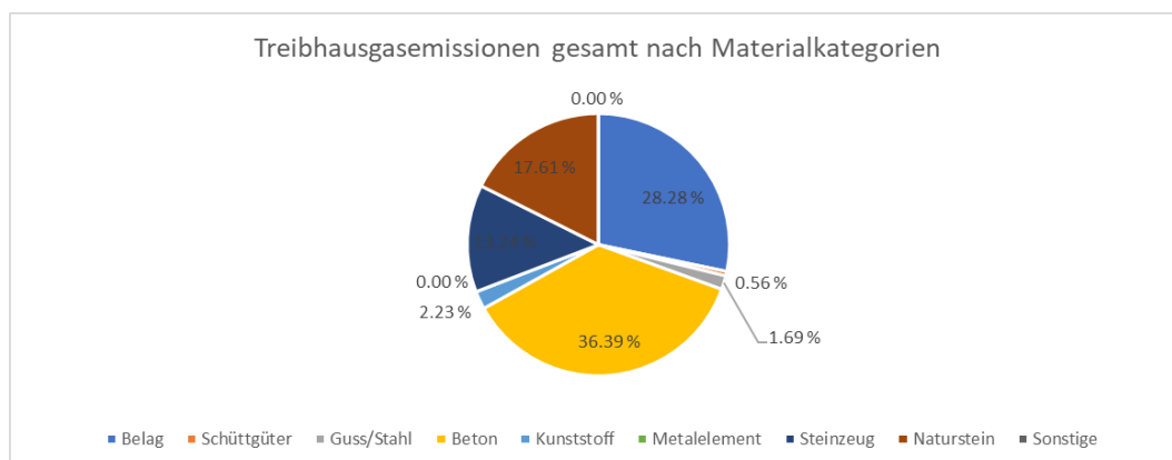
Abbildung 256: Winterthurerstrasse: Materialmengen nach Materialkategorien: Belag (Asphalt), Schüttgüter (Kiessande und Aushub), Guss/Stahl (Schachtdeckel und Schienen), Beton, Kunststoff (Rohre), Metalelemente (nur bei Sonderbauwerken), Steinzeug (Rohre), Naturstein (Randsteine und Pflasterung) und sonstige.
