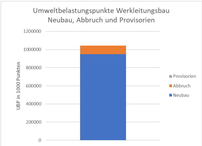
Abbildung 15: Allenmoosstrasse Werkleitungen: Umweltbelastungspunkte Neubau, Abbruch und Provisorien
