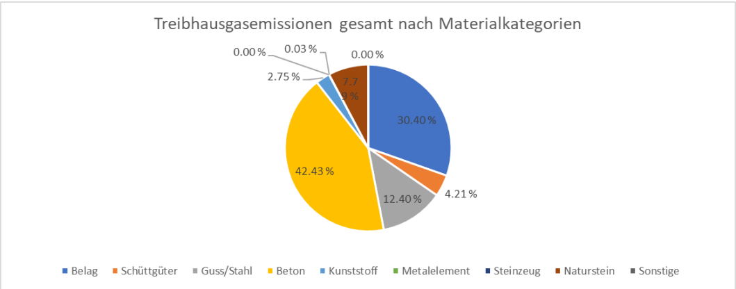
Abbildung 17: Gloriastrasse: Treibhausgasemissionen nach Materialkategorien: Belag (Asphalt), Schüttgüter (Kiessande und Aushub), Guss/Stahl (Schachtdeckel und Schienen), Beton, Kunststoff (Rohre), Metalelemente (nur bei Sonderbauwerken), Steinzeug (Rohre), Naturstein (Randsteine und Pflästerung) und sonstige.
