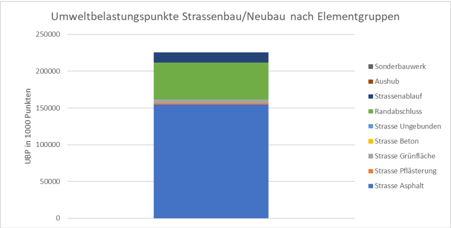
Abbildung 11: Allenmoosstrasse Strassenbau: Umweltbelastungspunkte des Neubaus unterschieden nach Elementgruppen
