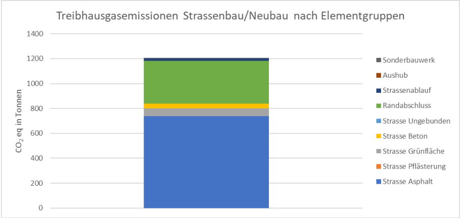
Abbildung 223: Witikonerstrasse: Treibhausgasemissionen des Neubaus unterschieden nach Elementgruppen
