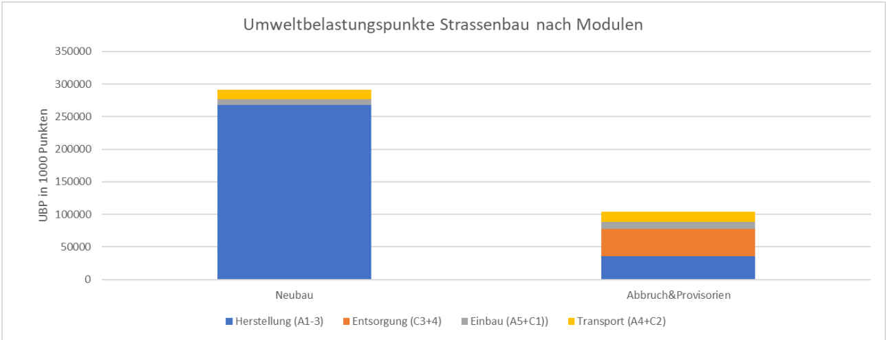
Abbildung 247: Universitätsstrasse: Umweltbelastungspunkte unterschieden nach Modulen
