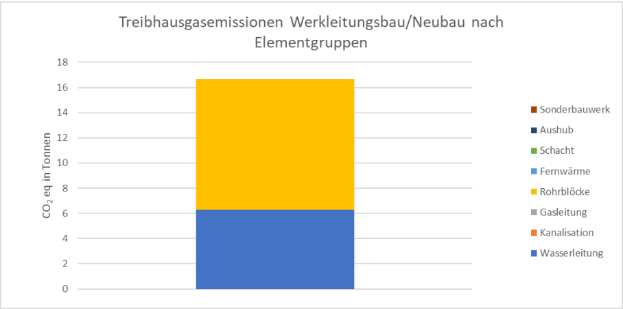
Abbildung 25: Gloriastrasse Werkleitungen: Treibhausgasemissionen des Neubaus unterschieden nach Elementgruppen
