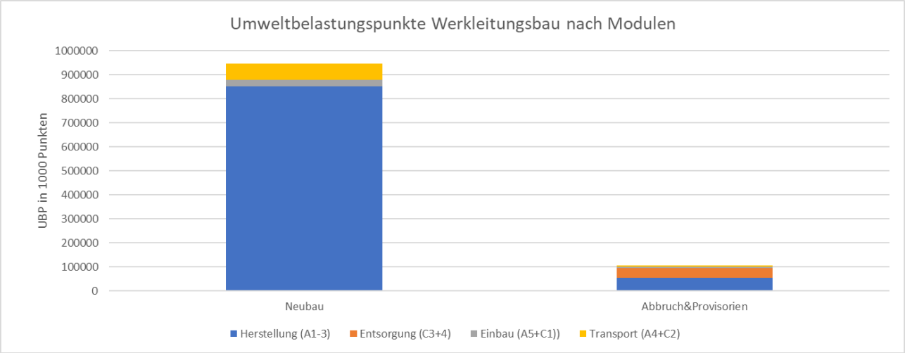
Abbildung 127: Rain Morgenstrasse Werkleitungen:Umweltbelastungspunkte unterschieden nach Modulen
