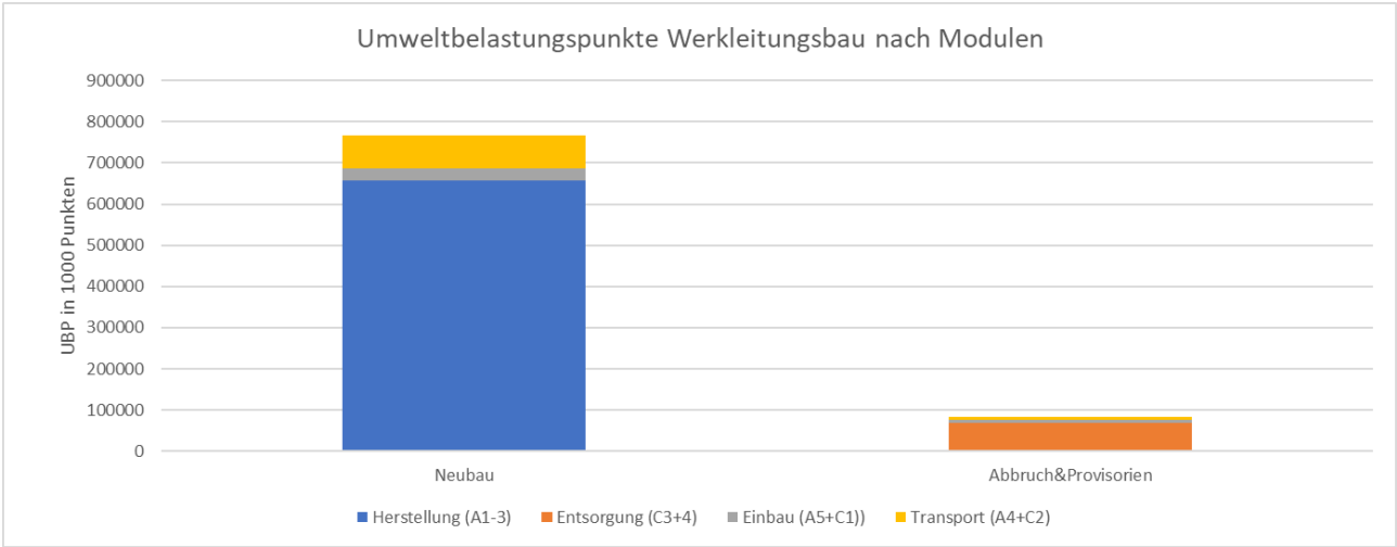
Abbildung 217: Wiesliacher Trichtenstrasse Werkleitungen:Umweltbelastungspunkte unterschieden nach Modulen
