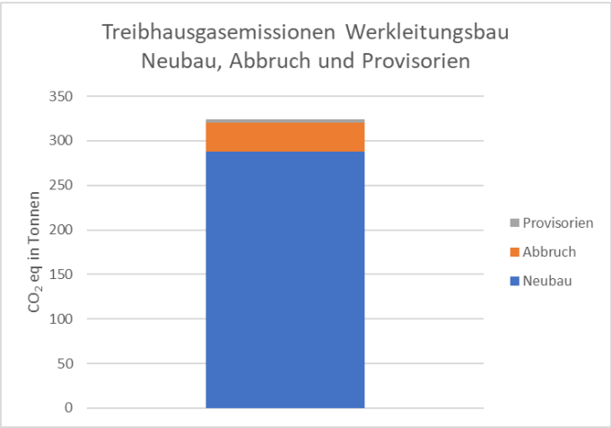
Abbildung 182: Sempacherstrasse Werkleitungen: Treibhausgasemissionen Neubau, Abbruch und Provisorien
