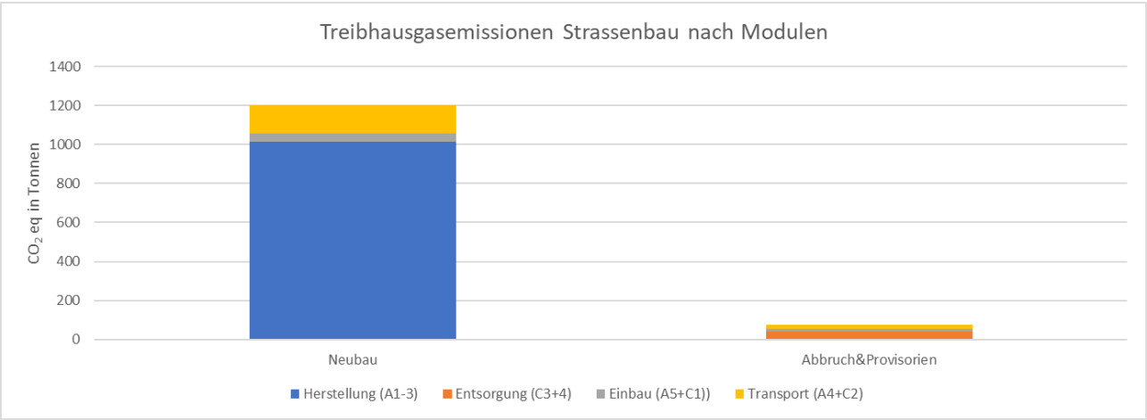
Abbildung 222: Witikonerstrasse: Treibhausgasemissionen unterschieden nach Modulen
