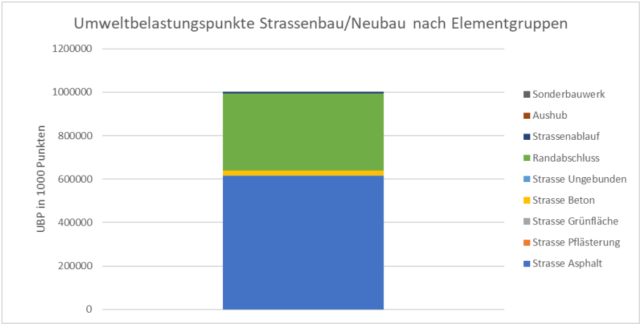
Abbildung 80: Manessestrasse Strassenbau: Umweltbelastungspunkte des Neubaus unterschieden nach Elementgruppen
