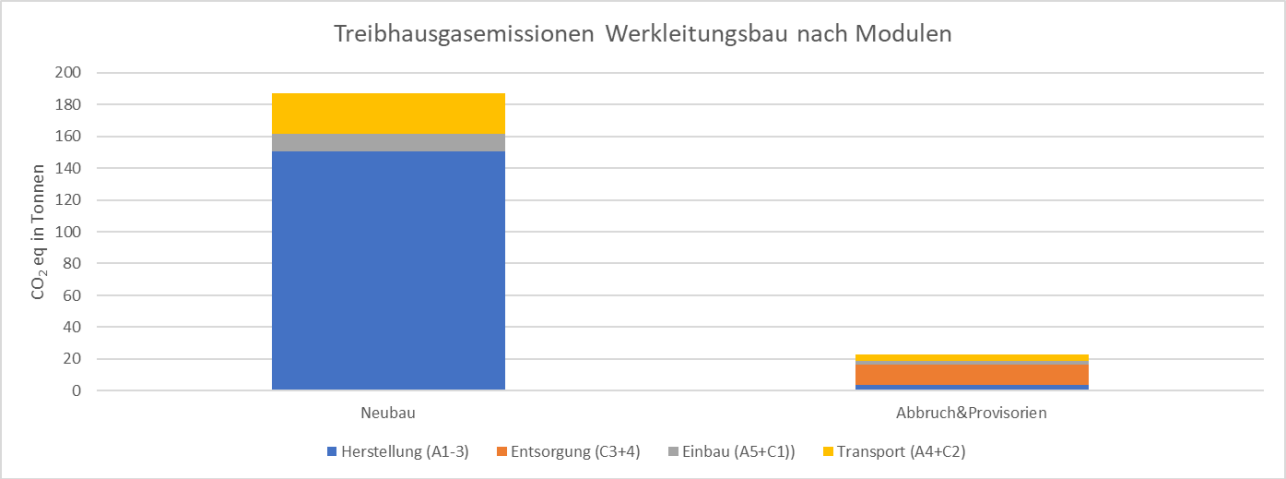
Abbildung 105: Mühlezellstrasse Werkleitungen: Treibhausgasemissionen unterschieden nach Modulen
