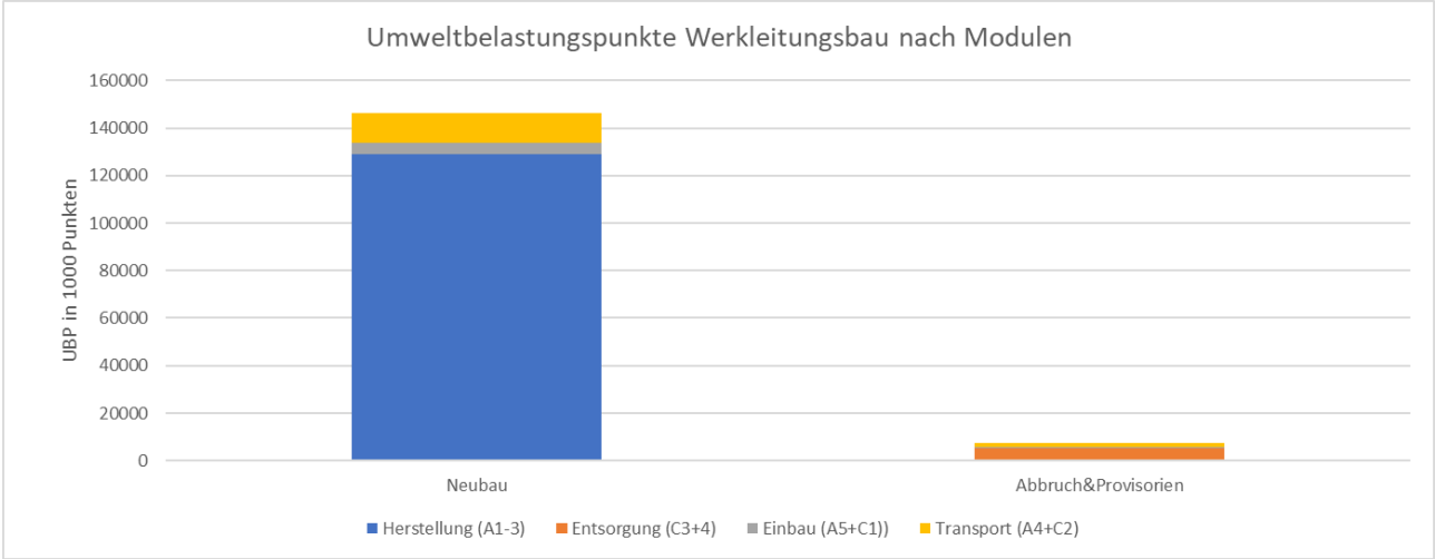
Abbildung 97: Marktplatz Oerlikon Werkleitungen:Umweltbelastungspunkte unterschieden nach Modulen
