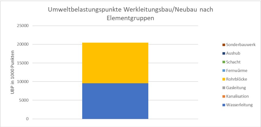
Abbildung 35: Glorიაstrasse Werkleitungen: Umweltbelastungspunkte des Neubaus unterschieden nach Elementgruppen
