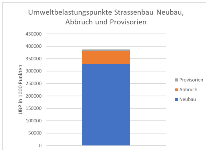
Abbildung 171: Saumstrasse Strassenbau: Umweltbelastungspunkte Neubau, Abbruch und Provisorien
