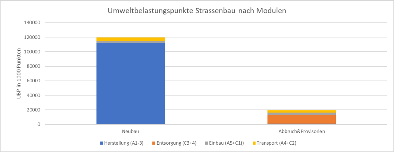
Abbildung 265: Winterthurerstrasse: Umweltbelastungspunkte unterschieden nach Modulen
