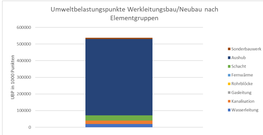
Abbildung 68: In der Ey Werkleitungen: Umweltbelastungspunkte des Neubaus unterschieden nach Elementgruppen
