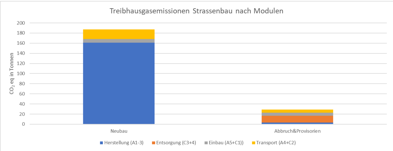
Abbildung 162: Saumstrasse: Treibhausgasemissionen unterschieden nach Modulen
