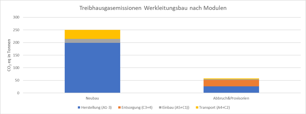
Abbildung 120: Rain Morgenstrasse Werkleitungen:Treibhausgasemissionen unterschieden nach Modulen
