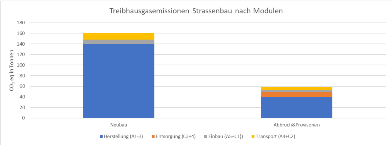
Abbildung 18: Gloriastrasse Strassenbau: Treibhausgasemissionen unterschieden nach Modulen
