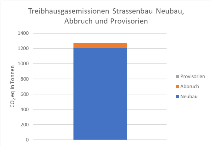
Abbildung 224: Witikonerstrasse Strassenbau: Treibhausgasemissionen Neubau, Abbruch und Provisorien
