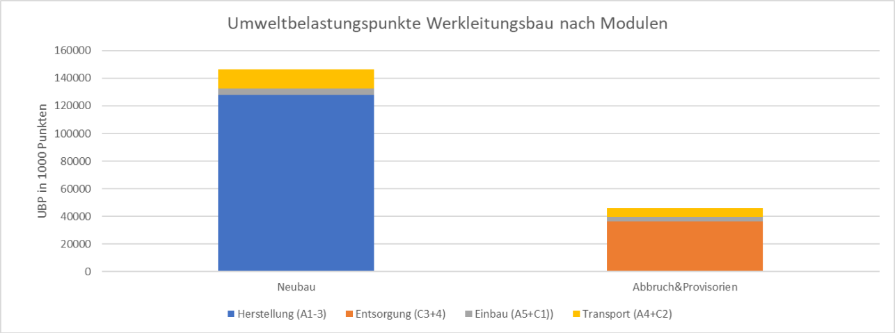
Abbildung 202: Sihlfeld Ernastrasse Werkleitungen:Umweltbelastungspunkte unterschieden nach Modulen
