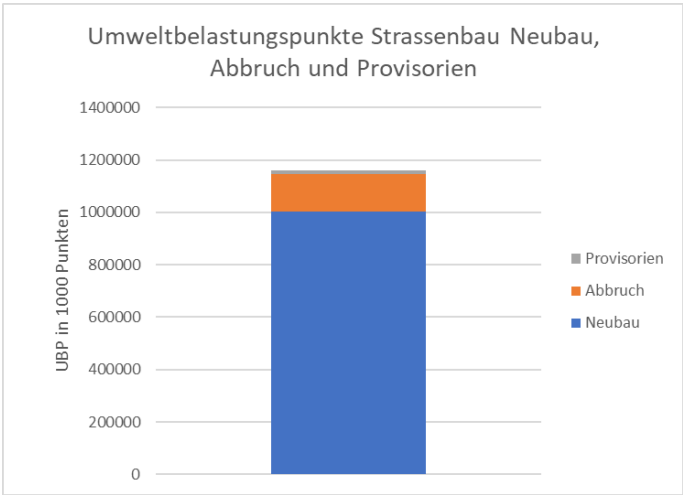
Abbildung 81: Manessestrasse Strassenbau: Umweltbelastungspunkte Neubau, Abbruch und Provisorien
