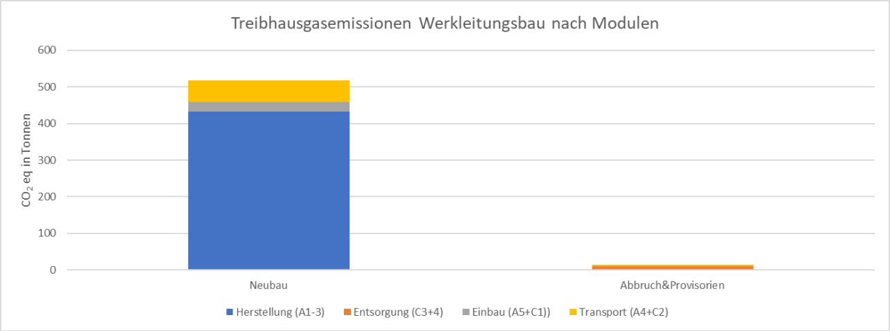
Abbildung 45: Haldenbach Werkleitungen: Treibhausgasemissionen unterschieden nach Modulen
