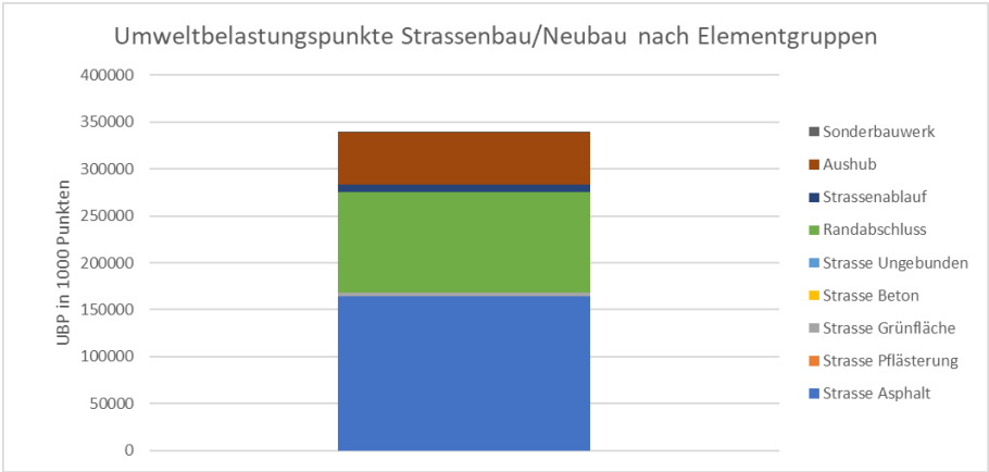
Abbildung 32: Gloriastrasse Strassenbau: Umweltbelastungspunkte des Neubaus unterschieden nach Elementgruppen
