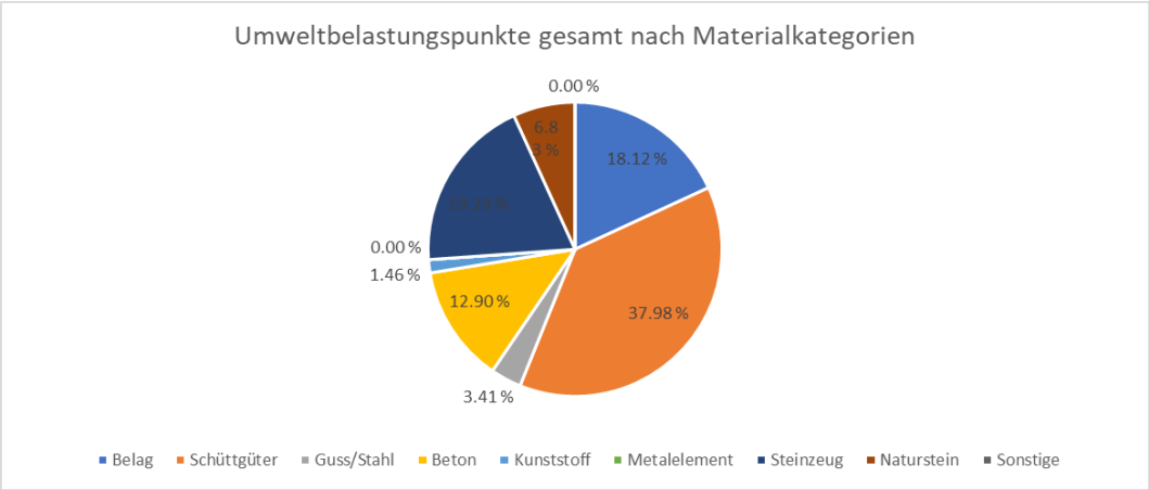
Abbildung 108: Mühlzellstrasse: Umweltbelastungspunkte nach Materialkategorien: Belag (Asphalt), Schüttgüter (Kiessande und Aushub), Guss/Stahl (Schachtdeckel und Schienen), Beton, Kunststoff (Rohre), Metalelemente (nur bei Sonderbauwerken), Steinzeug (Rohre), Naturstein (Randsteine und Pflästerung) und sonstige.
