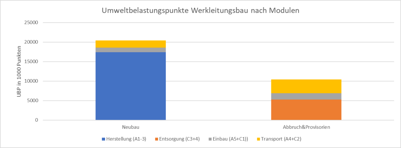
Abbildung 34: Glorიაstrasse Werkleitungen:Umweltbelastungspunkte unterschieden nach Modulen
