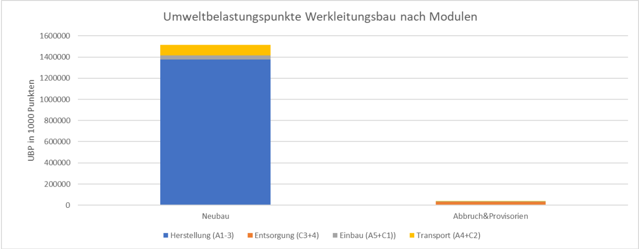
Abbildung 142: Regensbergstrasse Werkleitungen:Umweltbelastungspunkte unterschieden nach Modulen
