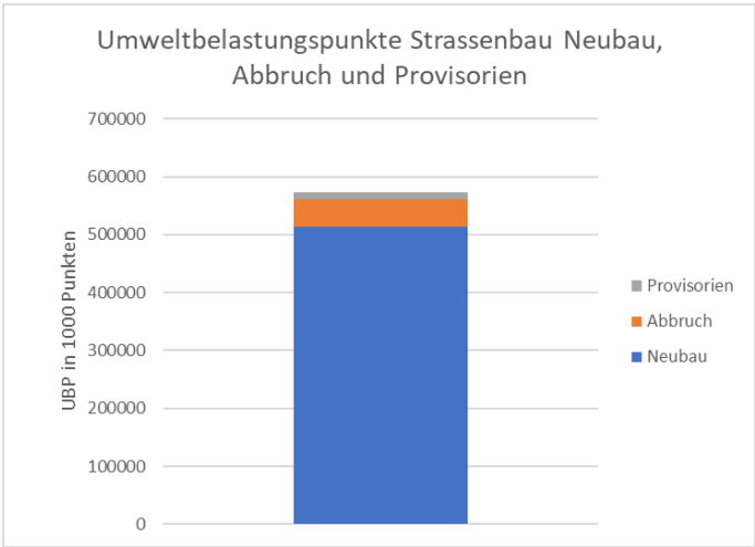
Abbildung 186: Sempacherstrasse Strassenbau: Umweltbelastungspunkte Neubau, Abbruch und Provisorien
