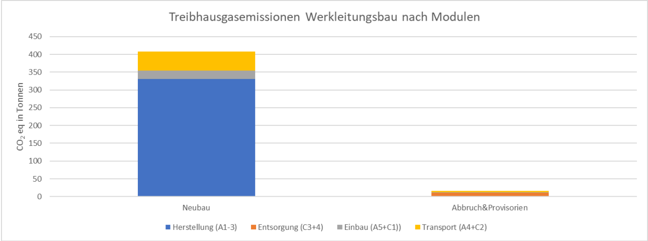
Abbildung 135: Regensbergstrasse Werkleitungen: Treibhausgasemissionen unterschieden nach Modulen
