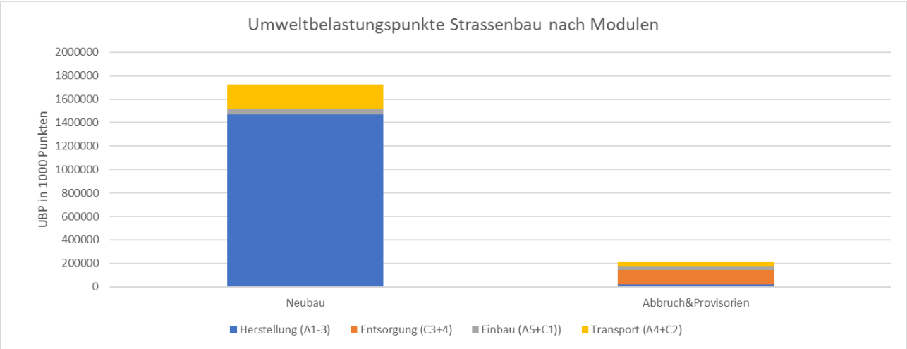
Abbildung 214: Wiesliacher Trichtenstrasse: Umweltbelastungspunkte unterschieden nach Modulen
