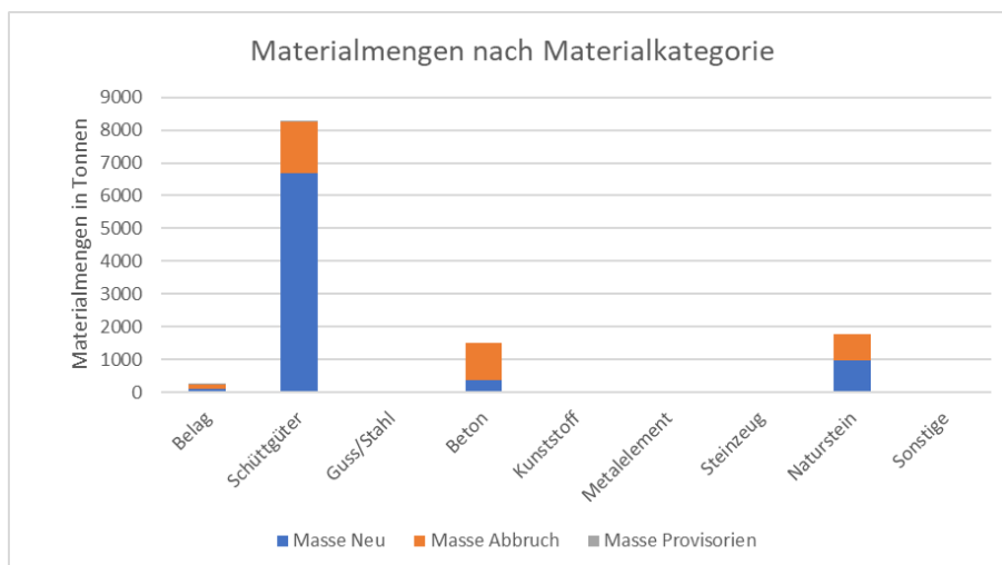
Abbildung 85: Marktplatz Oerlikon: Materialmengen nach Materialkategorien: Belag (Asphalt), Schüttgüter (Kiessande und Aushub), Guss/Stahl (Schachtdeckel und Schienen), Beton, Kunststoff (Rohre), Metallelemente (nur bei Sonderbauwerken), Steinzeug (Rohre), Naturstein (Randsteine und Pflasterung) und sonstige.
