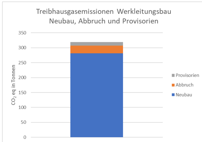
Abbildung 77: Manessestrasse Werkleitungen: Treibhausgasemissionen Neubau, Abbruch und Provisorien
