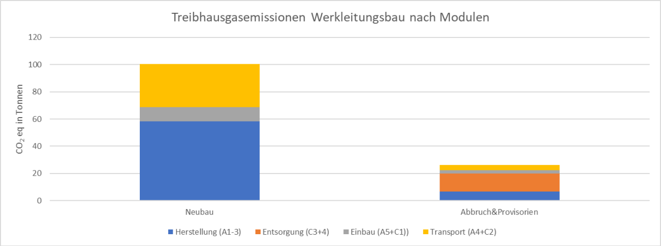
Abbildung 60: In der Ey Werkleitungen:Treibhausgasemissionen unterschieden nach Modulen
