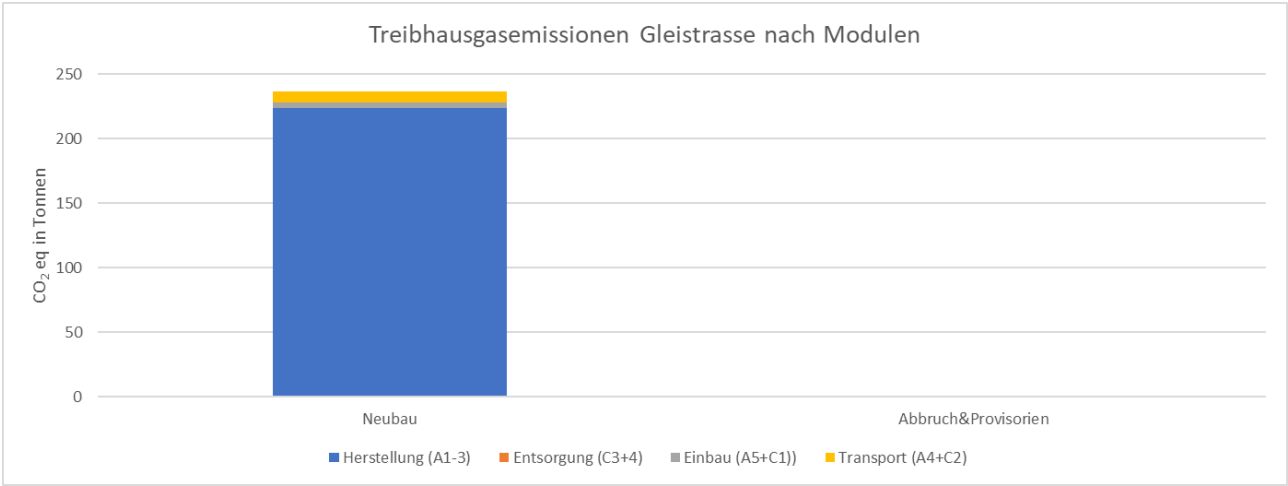
Abbildung 27: Glorიაstrasse Gleisbau: Treibhausgasemissionen unterschieden nach Modulen
