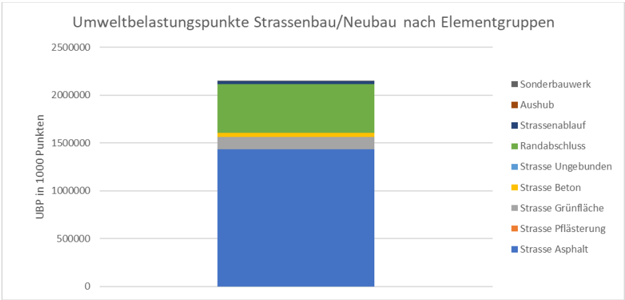
Abbildung 233: Witikonerstrasse Werkleitungen: Umweltbelastungspunkte des Neubaus unterschieden nach Elementgruppen
