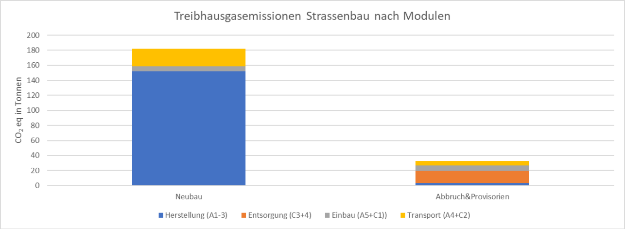
Abbildung 102: Mühlezellstrasse Strassenbau: Treibhausgasemissionen unterschieden nach Modulen
