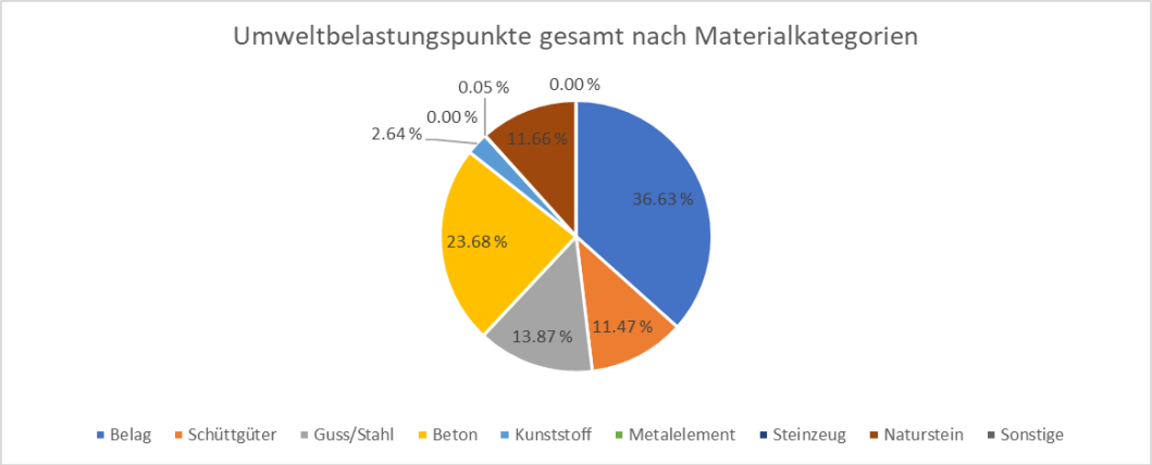
Abbildung 30: Gloristrasse: Umweltbelastungspunkte nach Materialkategorien: Belag (Asphalt), Schüttgüter (Kiessande und Aushub), Guss/Stahl (Schachtdeckel und Schienen), Beton, Kunststoff (Rohre), Metallelemente (nur bei Sonderbauwerken), Steinzeug (Rohre), Naturstein (Randsteine und Pflästerung) und sonstige.
