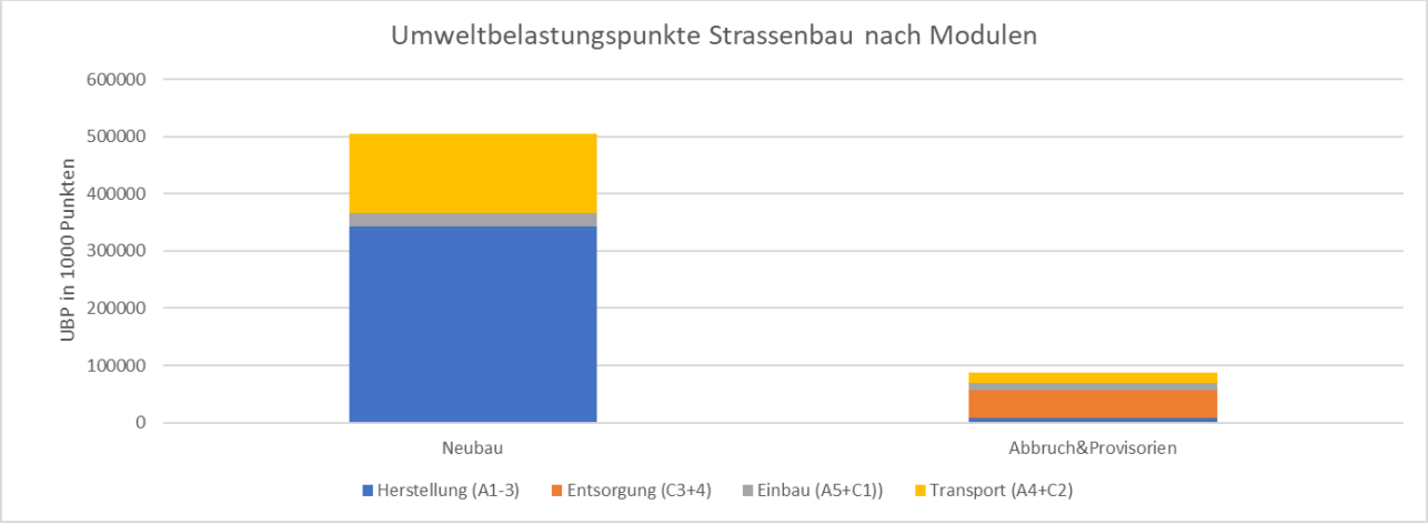
Abbildung 199: Sihlfeld Ernastrasse: Umweltbelastungspunkte unterschieden nach Modulen
