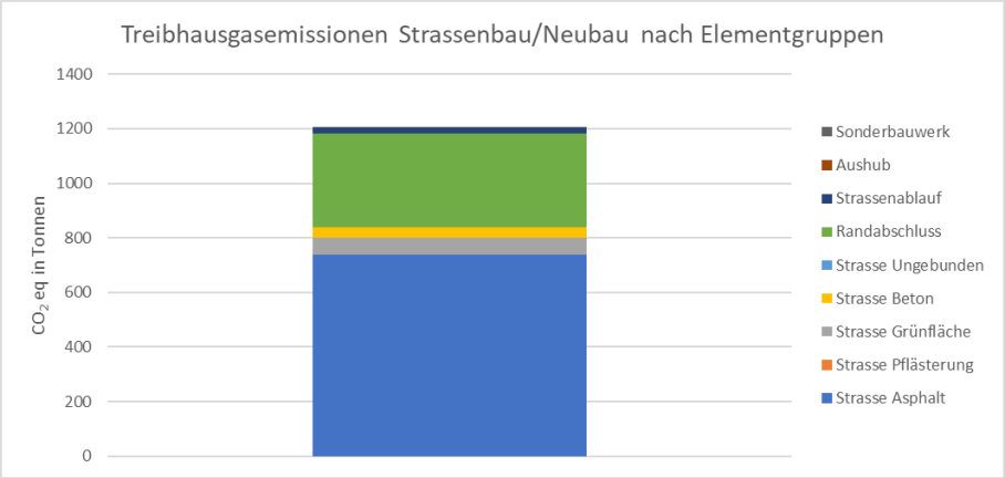
Abbildung 266: Winterthurerstrasse: Umweltbelastungspunkte des Neubaus unterschieden nach Elementgruppen
