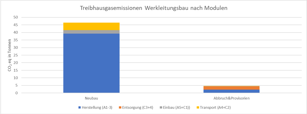
Abbildung 150: Rüdiger Staffel Werkleitungen: Treibhausgasemissionen unterschieden nach Modulen
