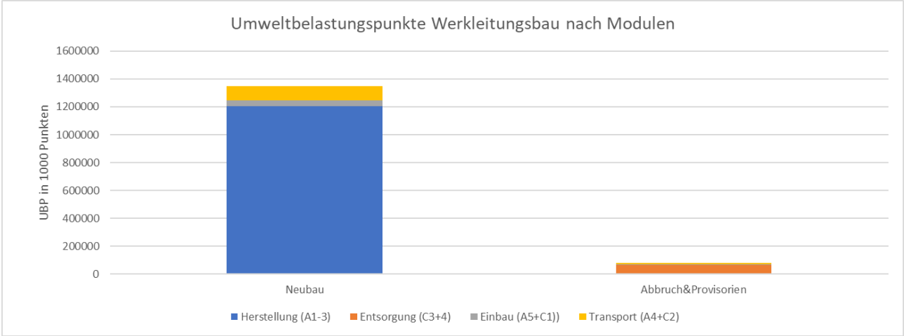
Abbildung 232: Witikonerstrasse Werkleitungen:Umweltbelastungspunkte unterschieden nach Modulen
