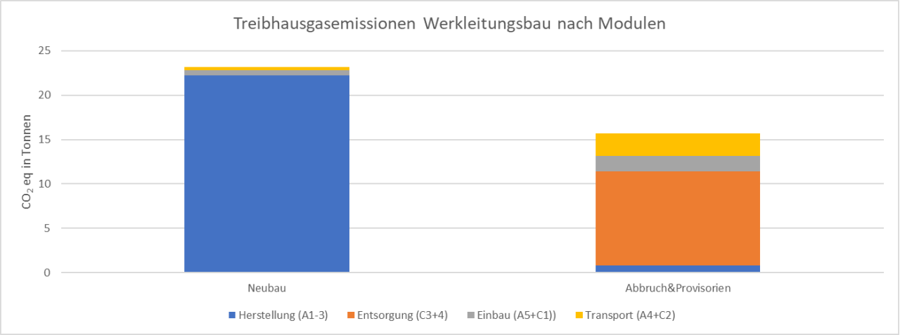
Abbildung 240: Universitätsstrasse Werkleitungen: Treibhausgasemissionen unterschieden nach Modulen
