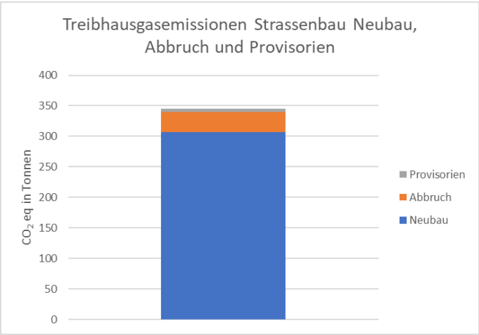
Abbildung 44: Haldenbach Strassenbau: Treibhausgasemissionen Neubau, Abbruch und Provisorien
