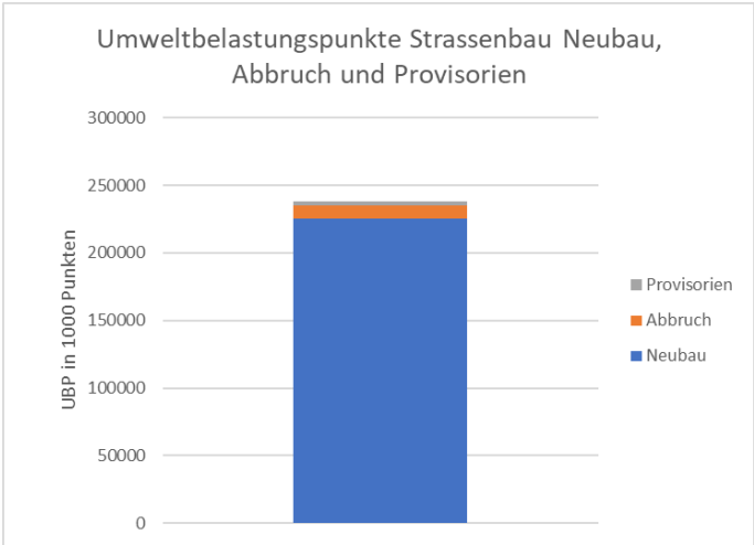
Abbildung 12: Allenmoosstrasse Strassenbau: Umweltbelastungspunkte Neubau, Abbruch und Provisorien
