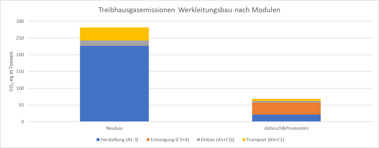
Abbildung 165: Saumstrasse Werkleitungen: Treibhausgasemissionen unterschieden nach Modulen
