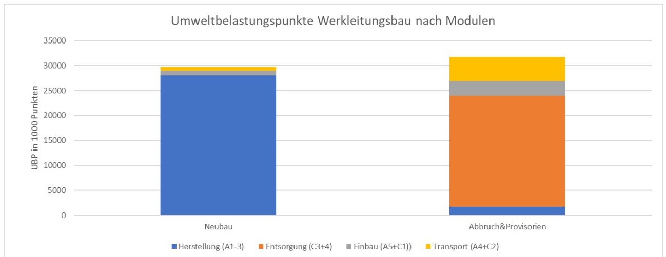
Abbildung 250: Universitätsstrasse Werkleitungen: Umweltbelastungspunkte unterschieden nach Modulen
