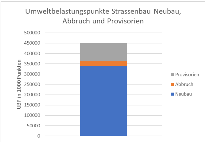
Abbildung 33: Gloriastrasse Strassenbau: Umweltbelastungspunkte Neubau, Abbruch und Provisorien
