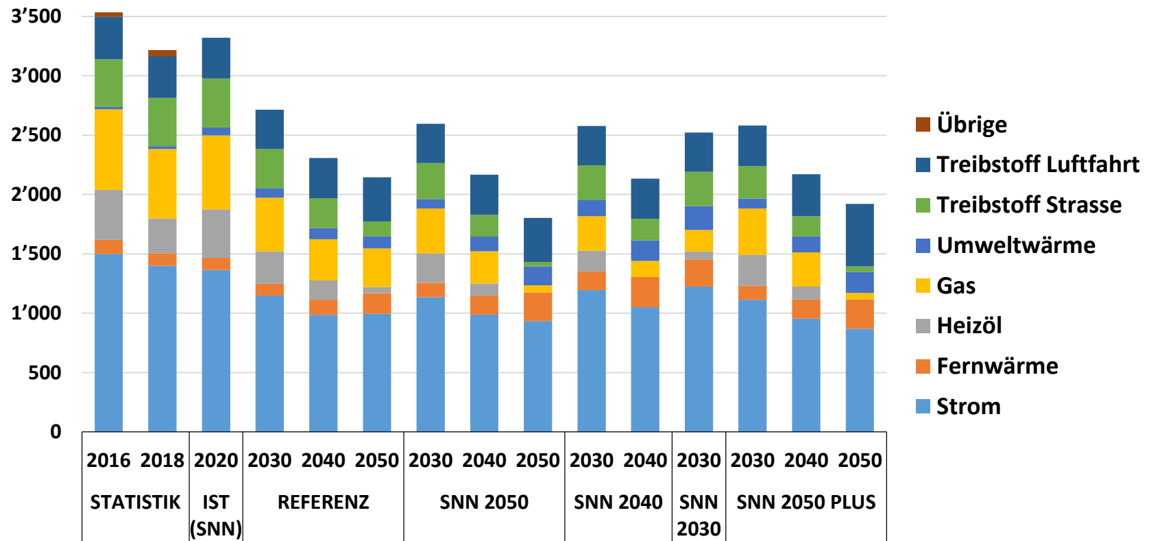
Dauerleistung W/Person
